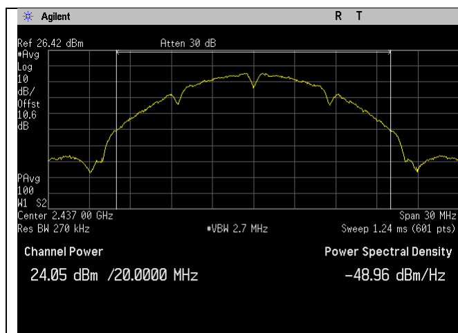
2437MHz_b-mode
