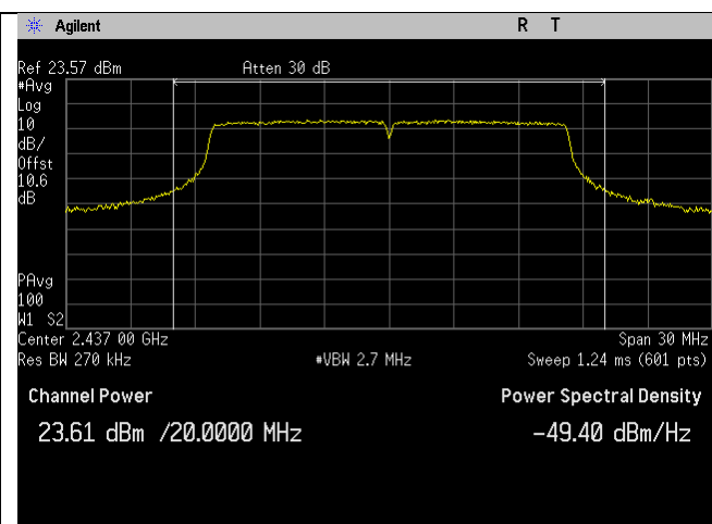
2437MHz_g-mode
