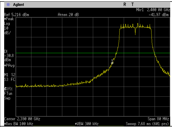
2412MHz_g-mode_Lower Band Edge
