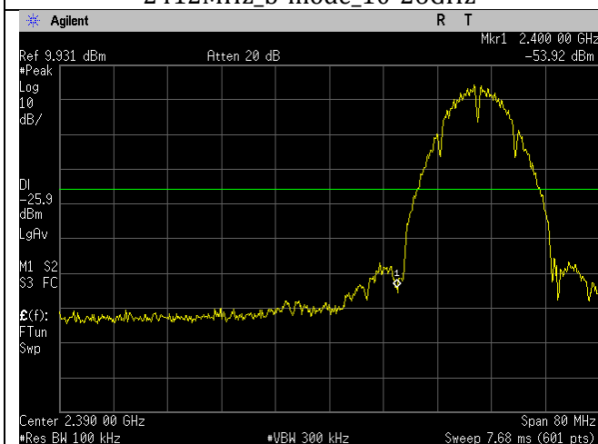
2412MHz_b-mode_Lower Band Edge
