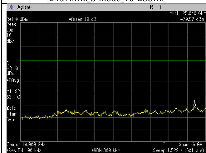
2437MHz_g-mode_10-26GHz
