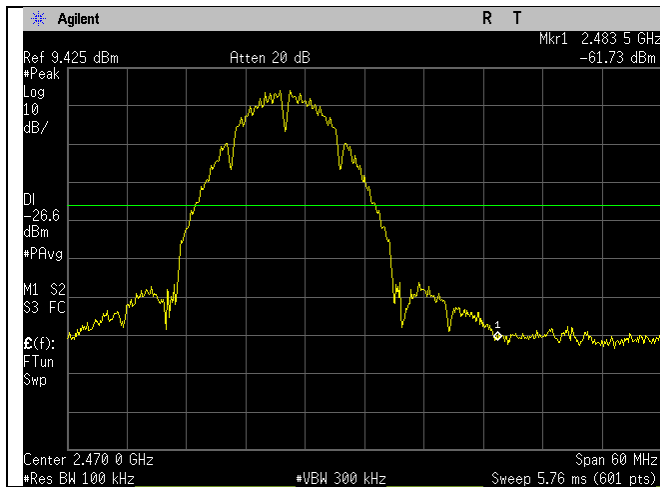
2462MHz_b-mode_Upper Band Edge
