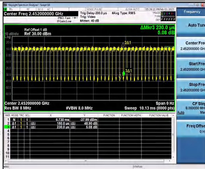
11AX40_Ant2_2452
