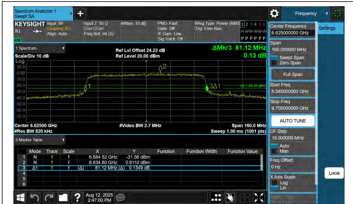
11AX80SISO-Ant2-6625
