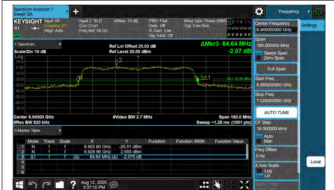
11AX80SISO-Ant1-7025
