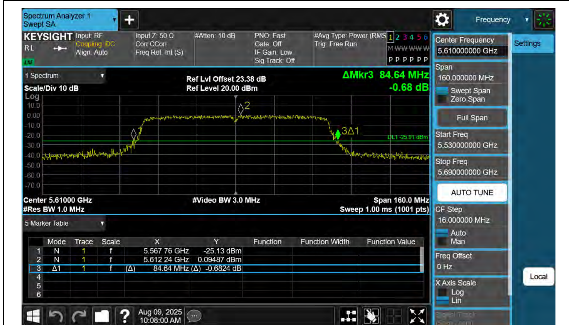
11AC80SISO-Ant2-5610
