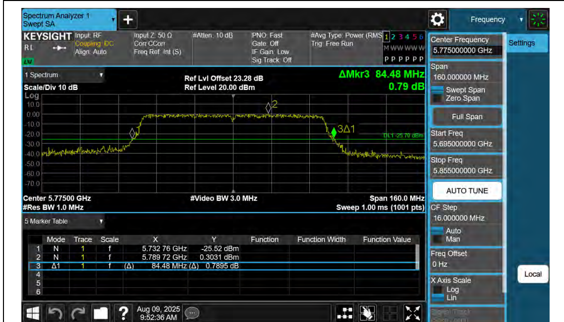
11AC80SISO-Ant2-5775
