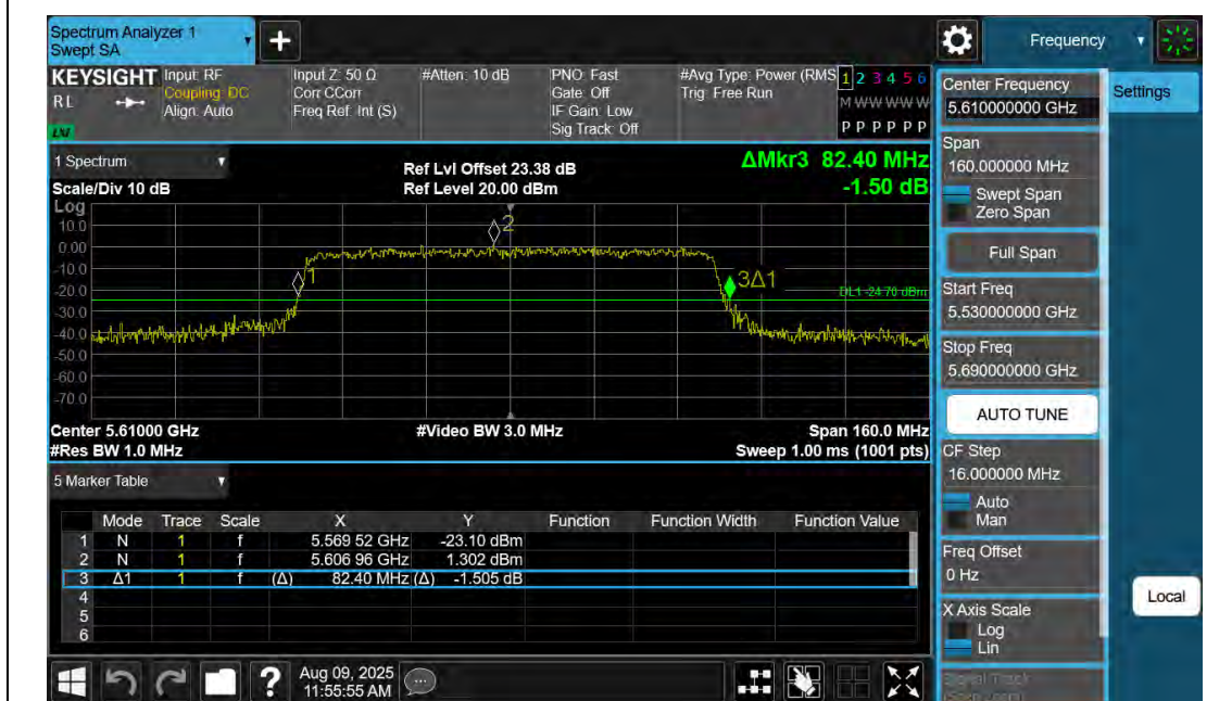
11AX80SISO-Ant2-5610
