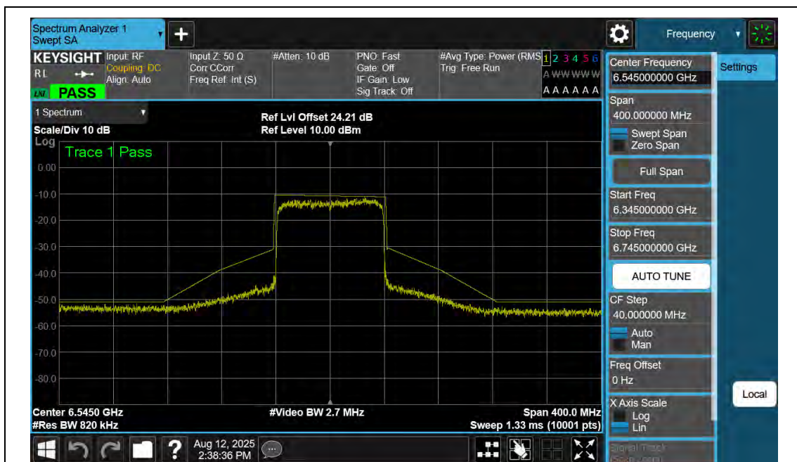
NTNV-11AX80SISO-Ant2-6545-PASS
