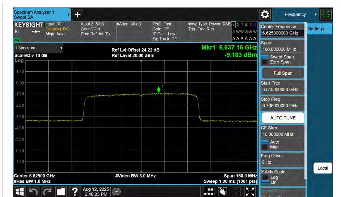
11AX80SISO-Ant2-6625-PASS
