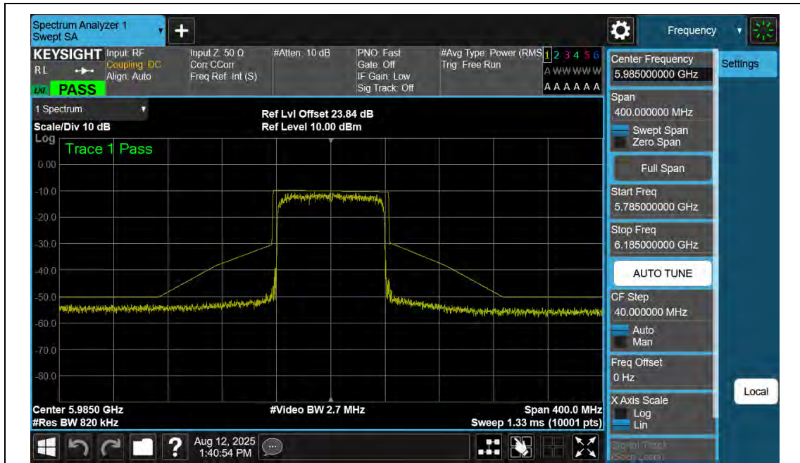
NTNV-11AX80SISO-Ant2-5985-PASS
