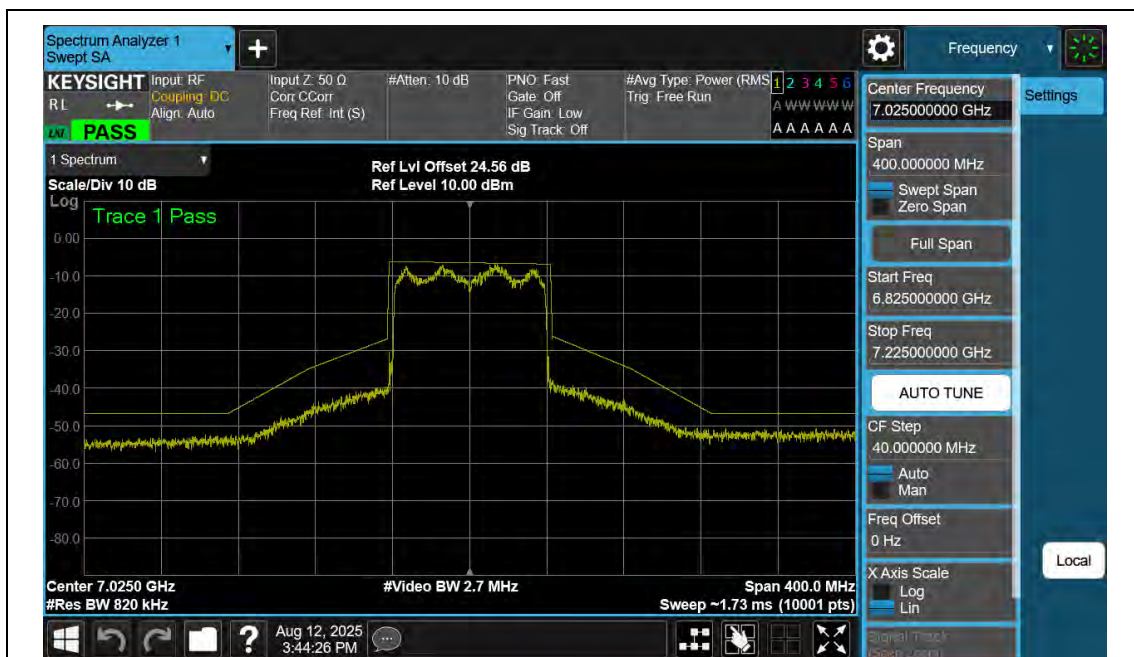
NTNV-11AX80SISO-Ant2-7025-PASS
