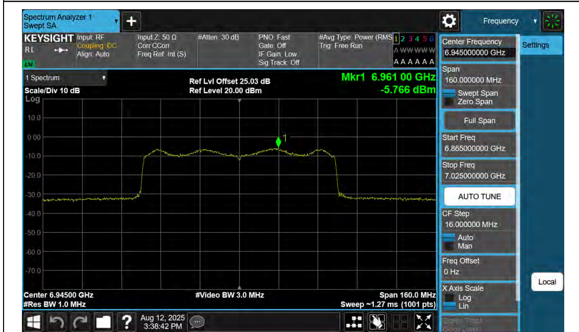
11AX80SISO-Ant1-7025-PASS
