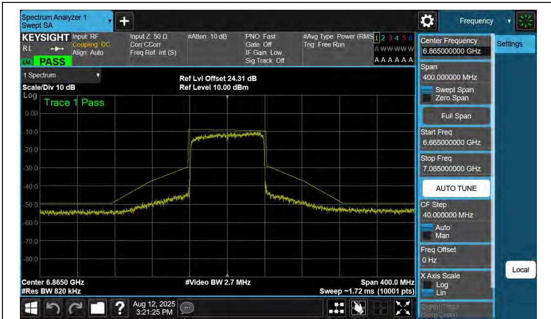
NTNV-11AX80SISO-Ant2-6865-PASS
