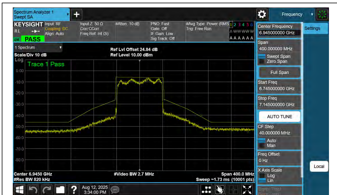
NTNV-11AX80SISO-Ant2-6945-PASS
