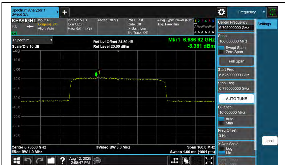
11AX80SISO-Ant2-6705-PASS
