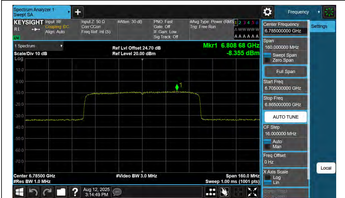
11AX80SISO-Ant1-6865-PASS
