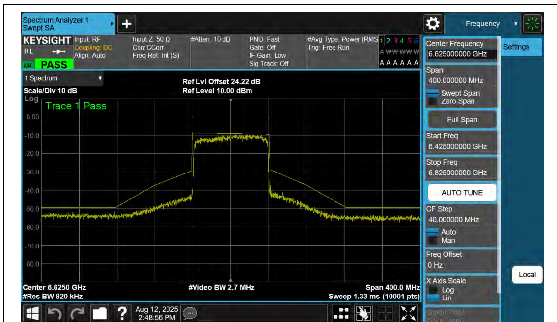
NTNV-11AX80SISO-Ant2-6625-PASS
