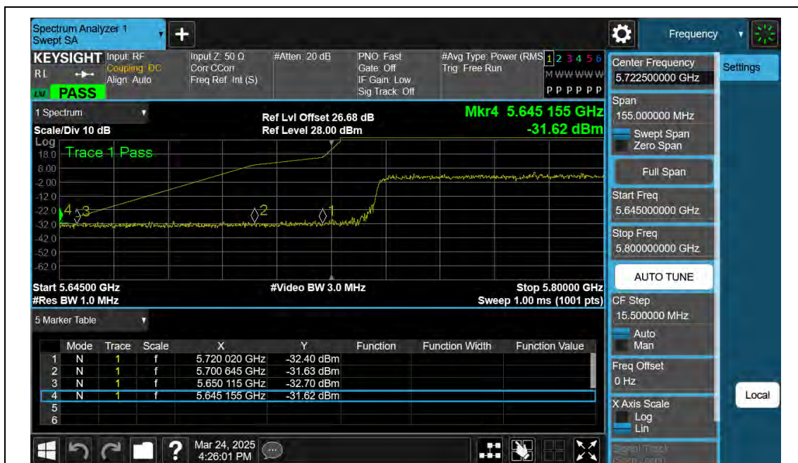
11AX80SISO-Ant1-5775-PASS
