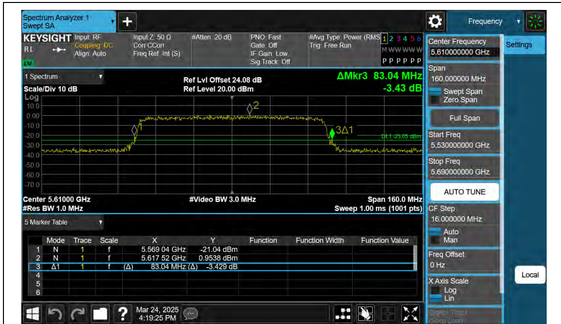
11AX80SISO-Ant2-5610
