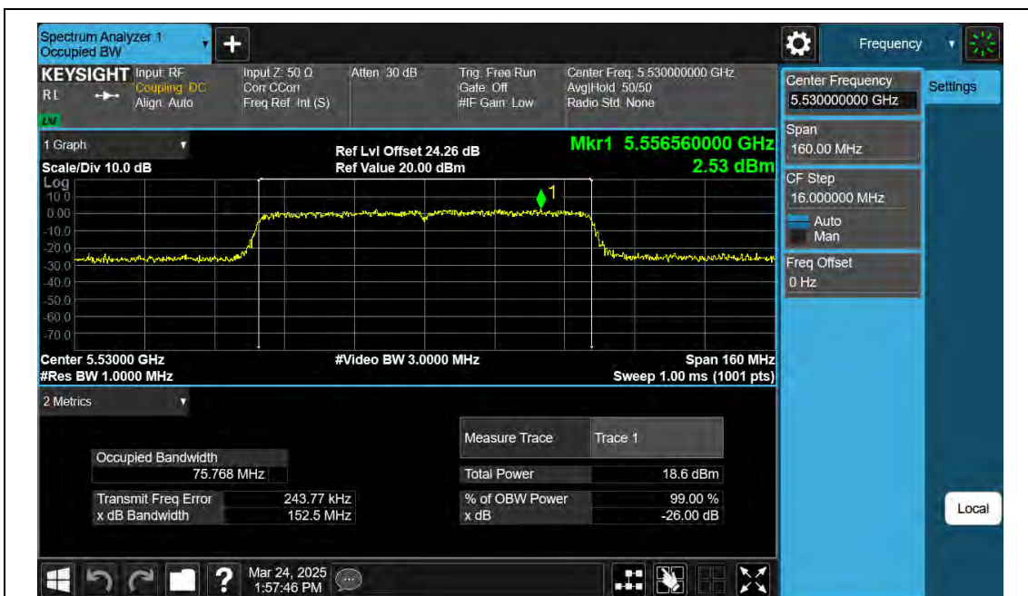
11AC80SISO-Ant2-5530
