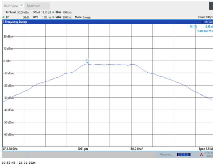
DH5_Ant1_2480
