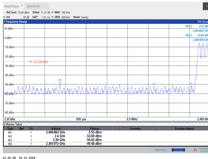
DH5_Ant1_Low_Hop_2402
