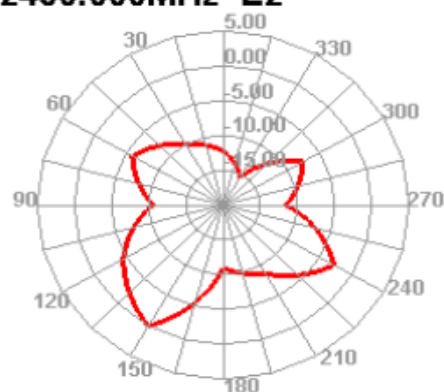
2450.000MHz E2
