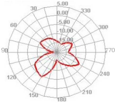
2500.000MHz E2
