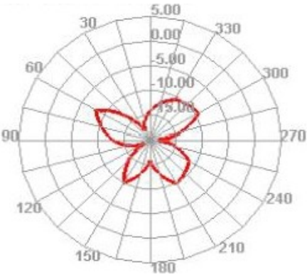
2500.000MHz E1
