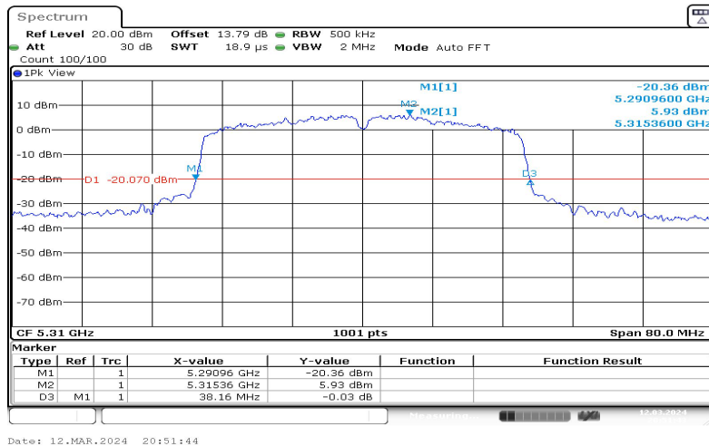
11N40SISO-Ant1-5310
