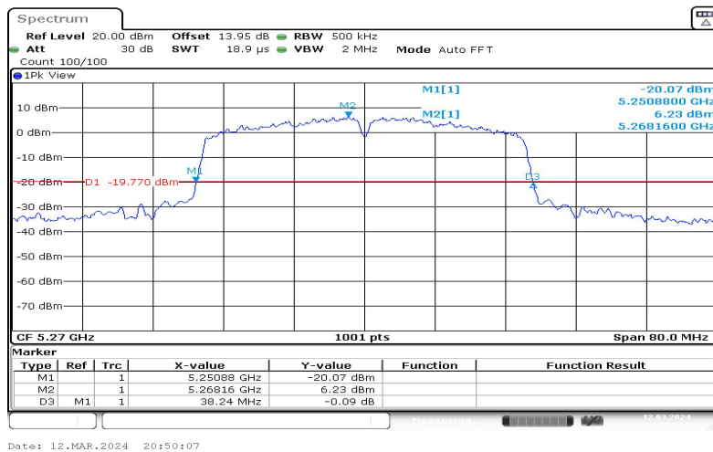
11N40SISO-Ant1-5270
