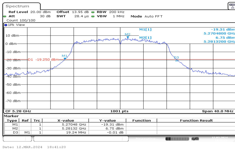
11A-Ant1-5280
