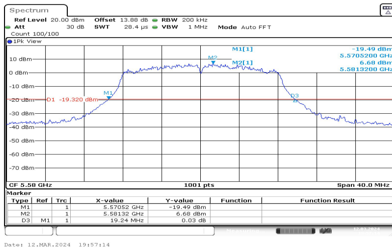
11A-Ant1-5580
