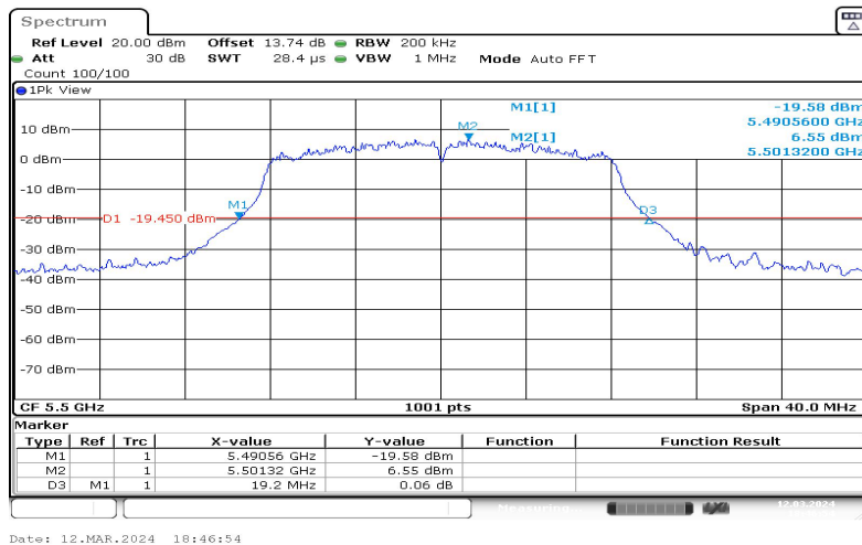
11A-Ant1-5500
