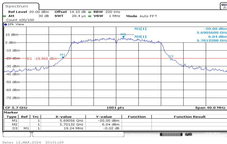
11A-Ant1-5700
