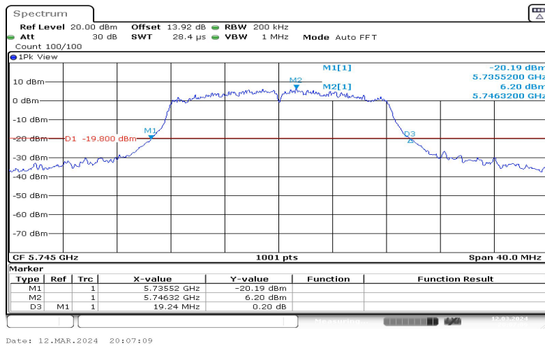
11A-Ant1-5745
