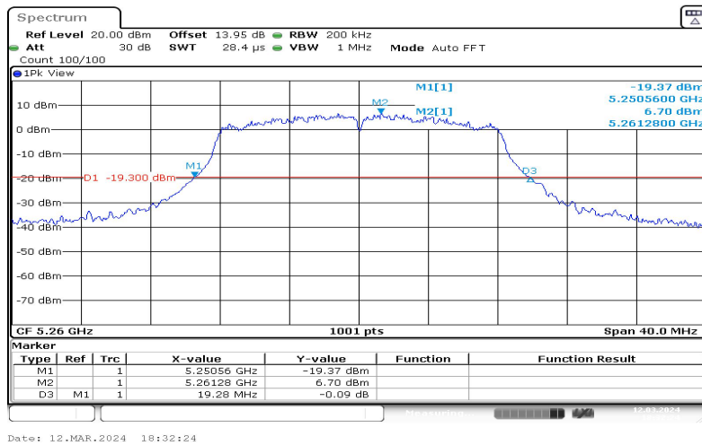
11A-Ant1-5260
