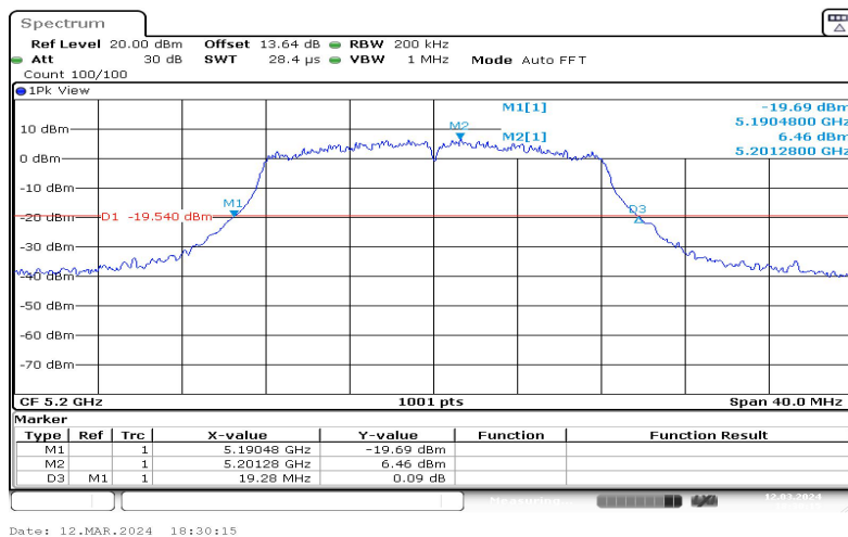
11A-Ant1-5200
