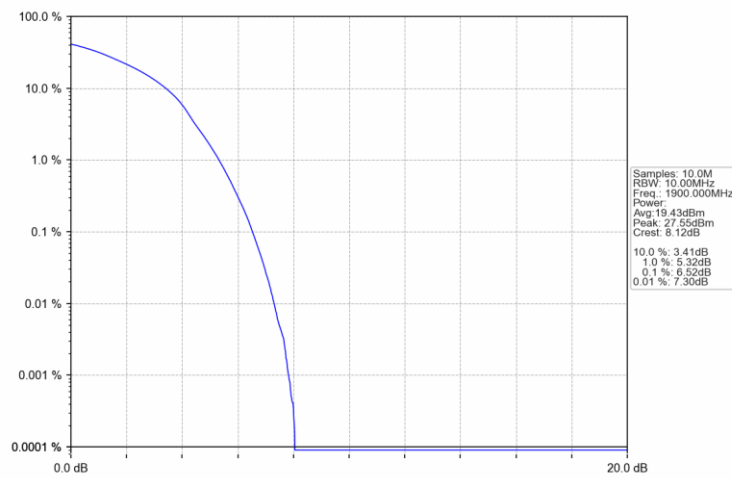
Band2_20MHz_16QAM_HCH_1900MHz_RB_100_0_NTNV
