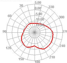
900.000MHz E1
