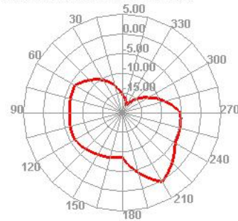
5900.000MHz Phi=45
