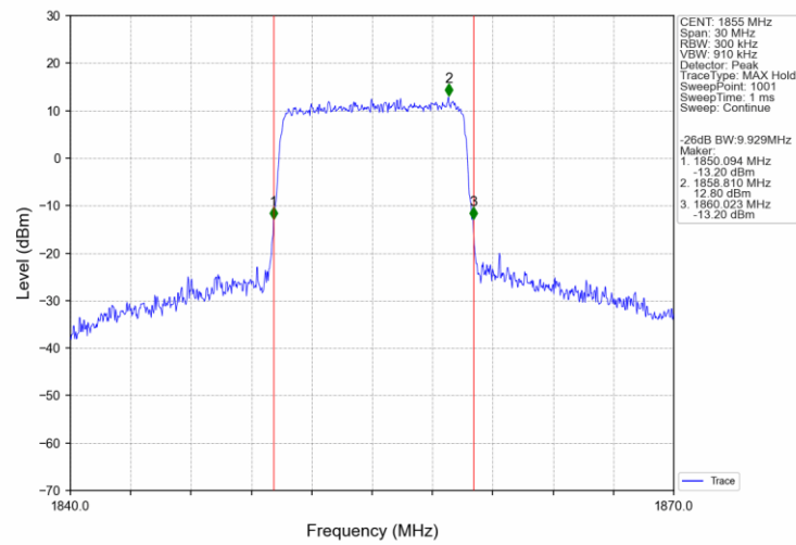
Band2 10MHz 16QAM LCH 1855MHz RB 50 0 NTN
