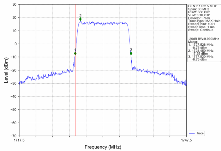
Band4 10MHz QPSK MCH 1732.5MHz RB 50 0 NTNV
