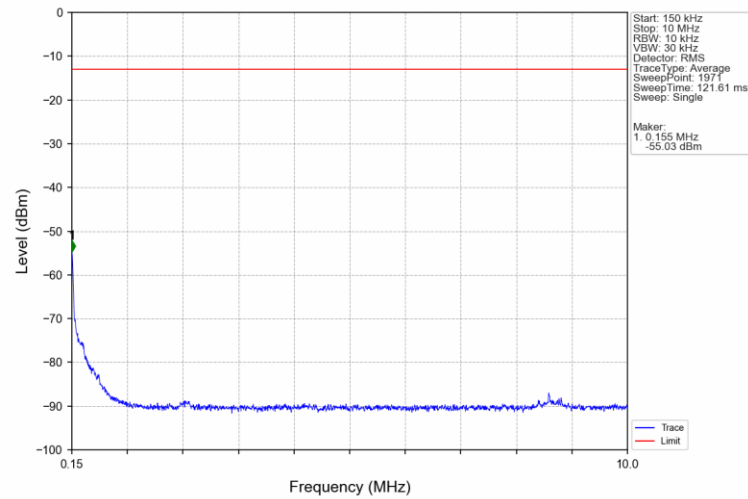
Band5 5MHz QPSK LCH 826.5MHz RB 1 0 NTNV
