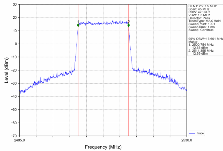
Band7 15MHz 16QAM LCH 2507.5MHz RB 75 0 NTNV
