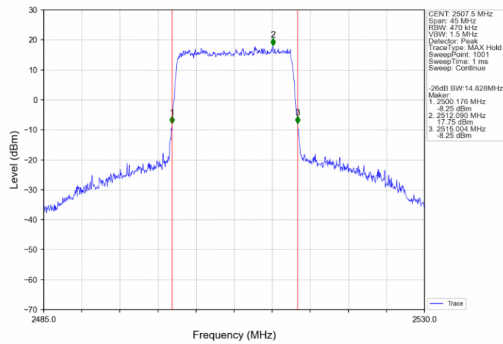
Band7 15MHz 16QAM LCH 2507.5MHz RB 75 0 NTNV
