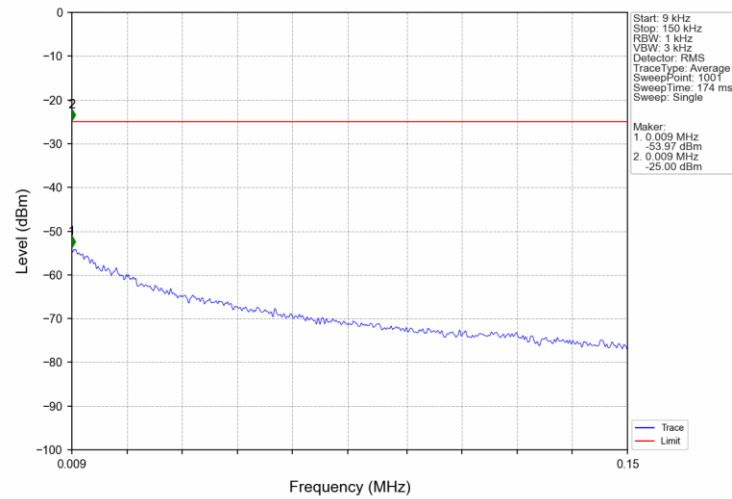
Band7 10MHz QPSK MCH 2535MHz RB 1 0 NTN
