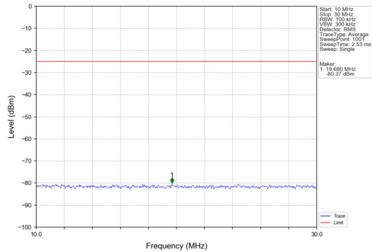
Band7 5MHz QPSK HCH 2567.5MHz RB 1 0 NTN
