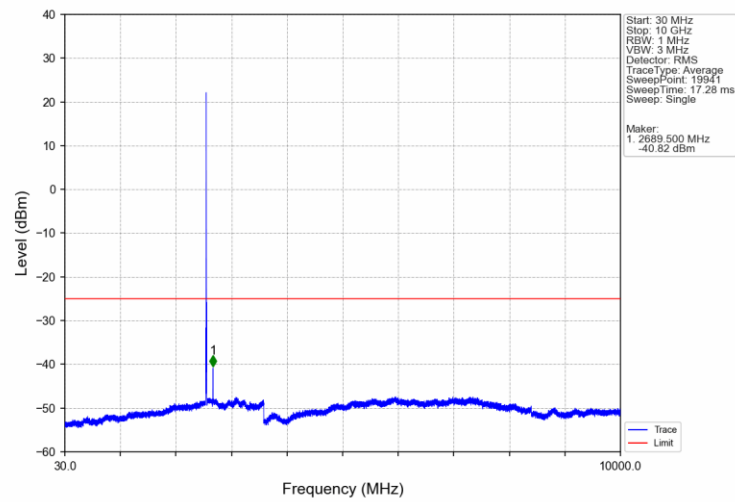
Band7 5MHz QPSK HCH 2567.5MHz RB 1 0 NTN
