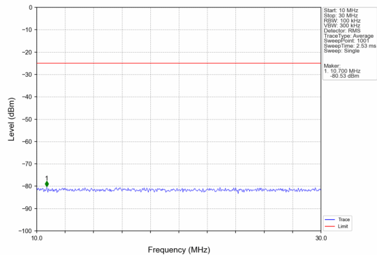
Band7 10MHz QPSK LCH 2505MHz RB 1 0 NTN
