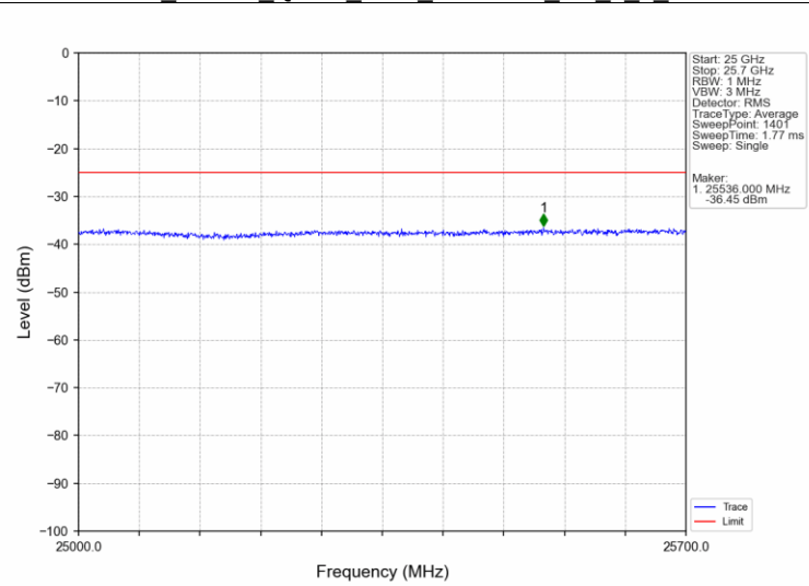
Band7 20MHz QPSK HCH 2560MHz RB 1 0 NTN
