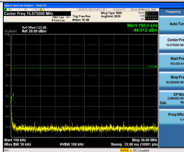
GSM850-251-0.15~30MHz
