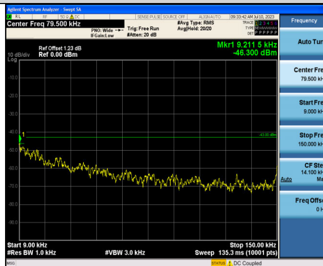
GSM1900-810-0.009~0.15MHz
