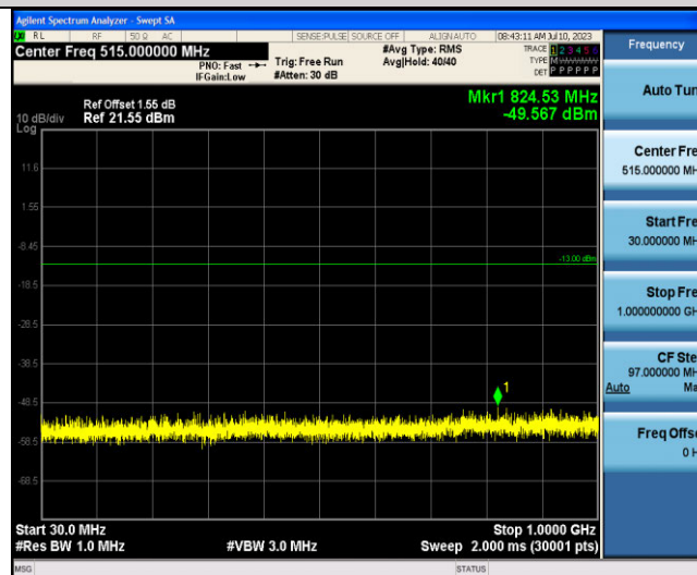
GPRS1900-661-30~1000MHz
