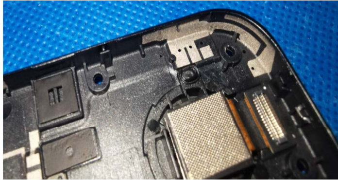
GPS/WIFI/BT antenna
