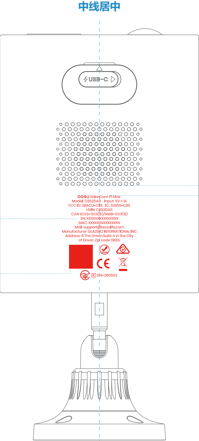
产品背面1:1尺寸线稿
