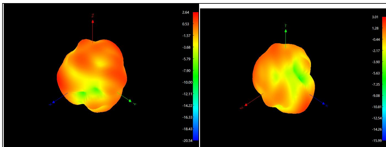
BT: 2450Mhz
