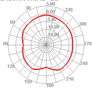
2420.000MHz E2
