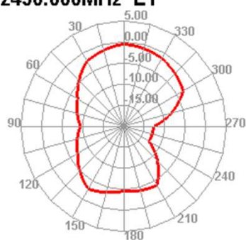
2450.000MHz E1
