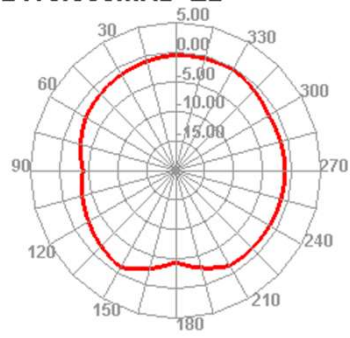
2460.000MHz E2
