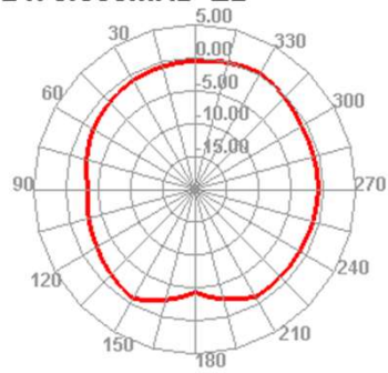
2480.000MHz H
