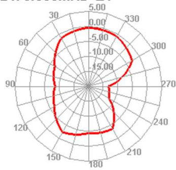
2480.000MHz
