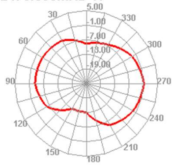
2470.000MHz H
