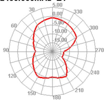
2440.000MHz
