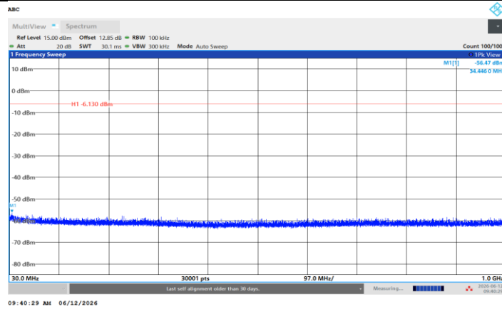
BLE 2M_Ant2_2478_30~1000
