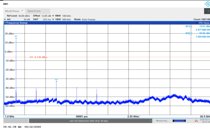
BLE 2M_Ant2_2478_1000~26500
