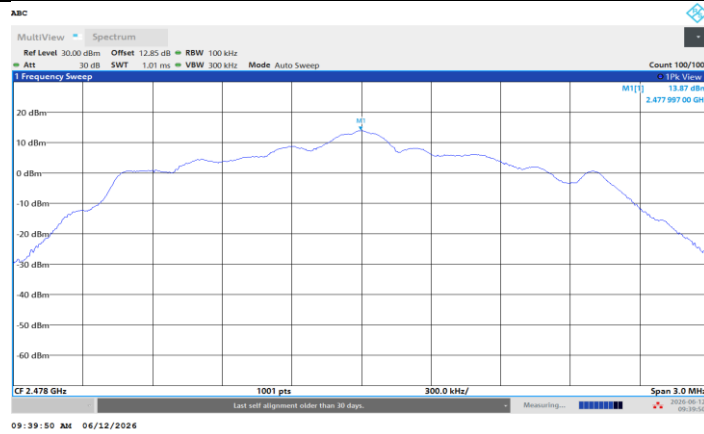
BLE 2M_Ant2_2478_0~Reference
