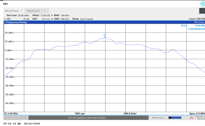
BLE 2M_Ant2_2440_0~Reference
