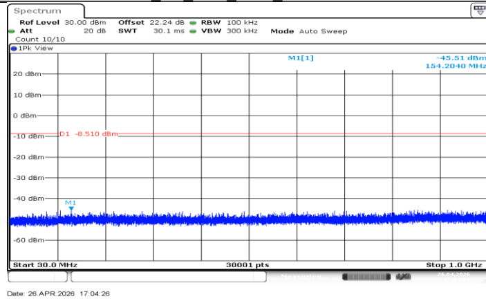
BLE_2M_Ant2_2402_30~1000
