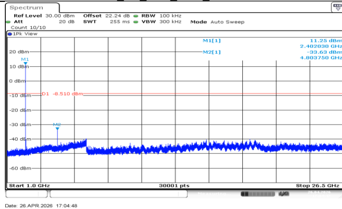
BLE_2M_Ant2_2402_1000~26500
