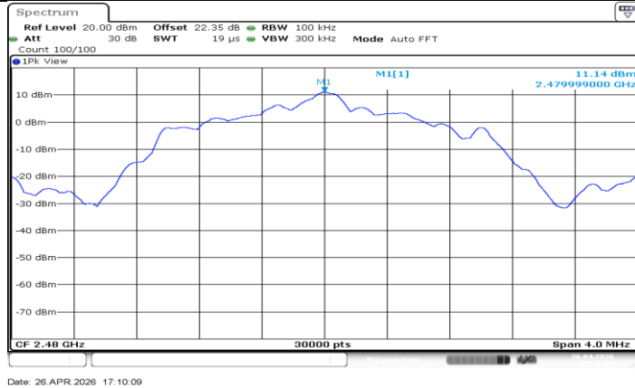
BLE_2M_Ant2_2480
