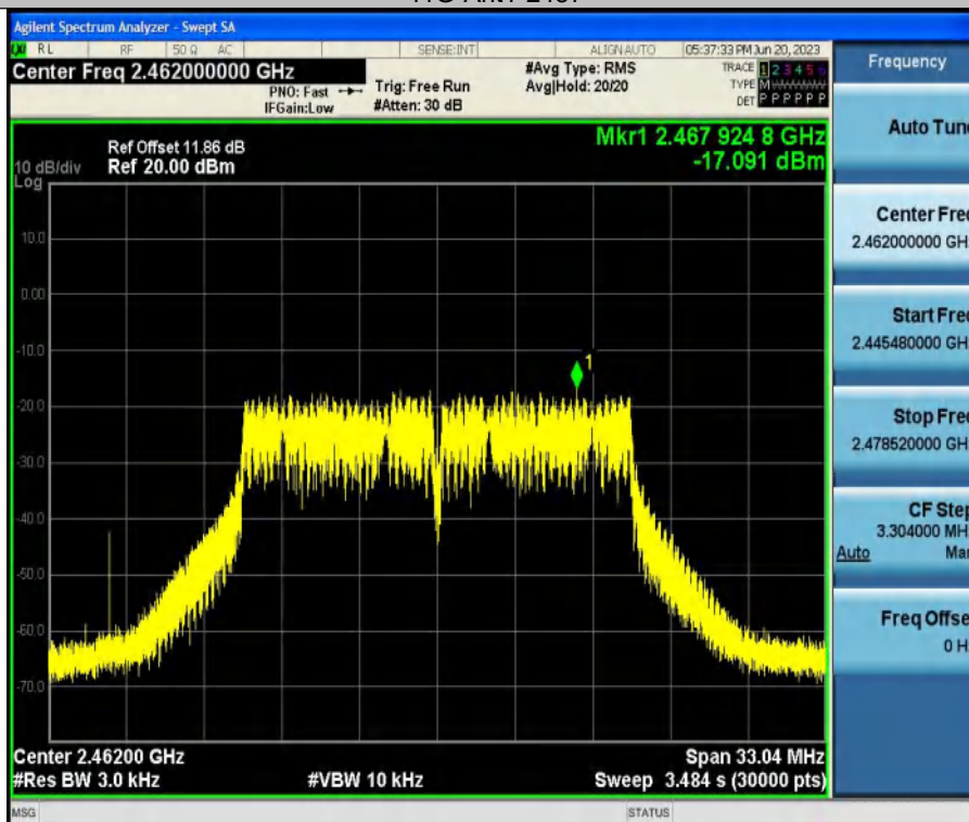
11G-Ant1-2462
