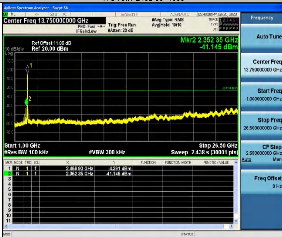
11G-Ant1-2462-1000~26500
