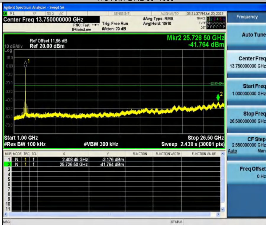
11G-Ant1-2412-1000~26500
