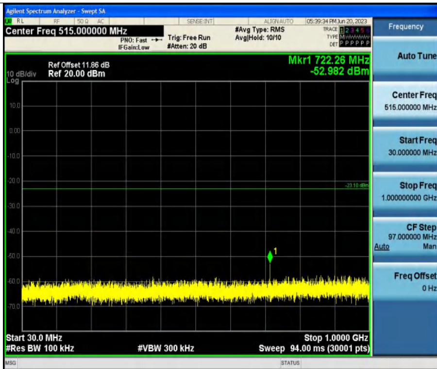
11G-Ant1-2462-30~1000
