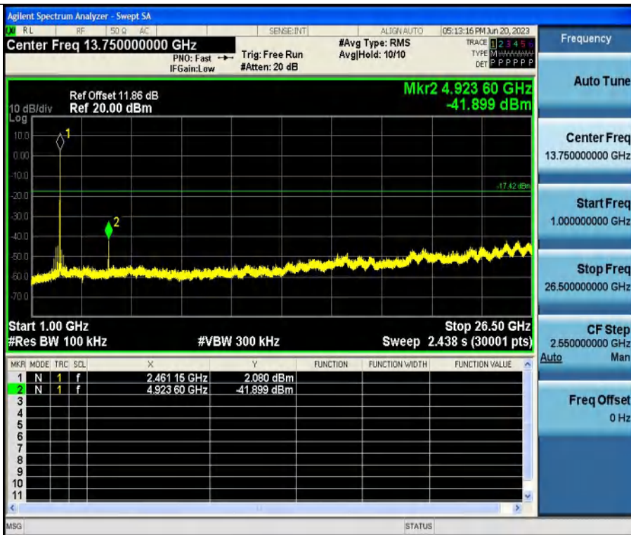
11B-Ant1-2462-1000~26500
