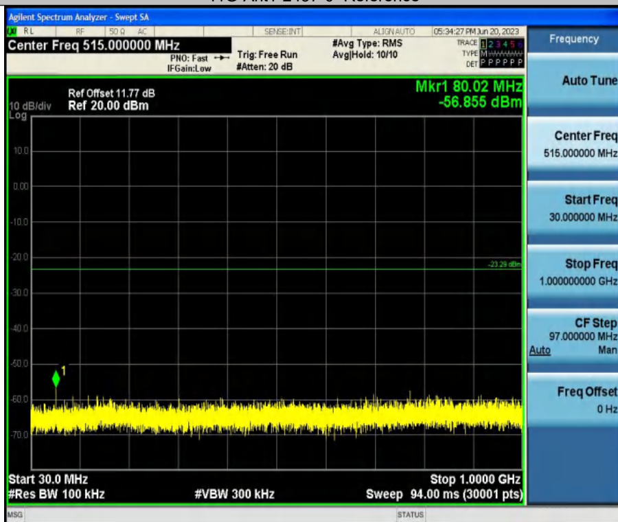
11G-Ant1-2437-30~1000
