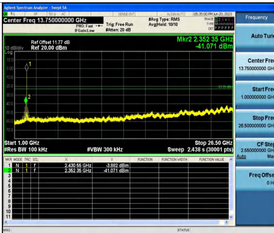
11G-Ant1-2437-1000~26500
