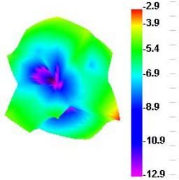
5150.000MHz
