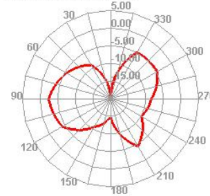
5490.000MHz E2
