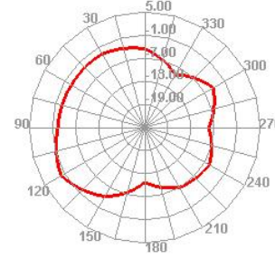
5490.000MHz E2
