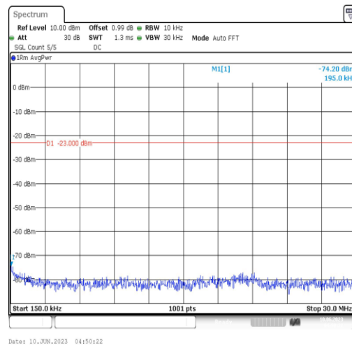
Band12-3MHz-QPSK-23095-1RB#0-Range2:0.15~30MHz
