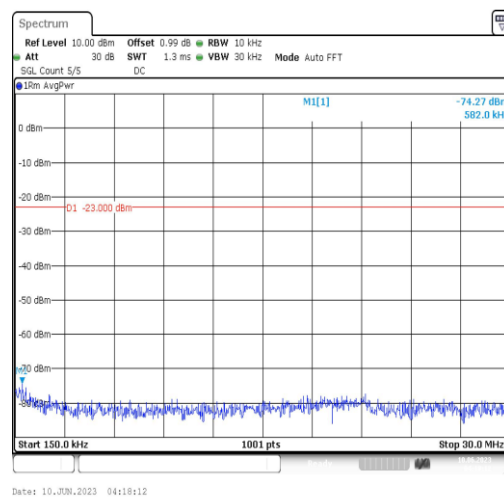
Band12-1.4MHz-QPSK-23095-1RB#0-Range2:0.15~30MHz
