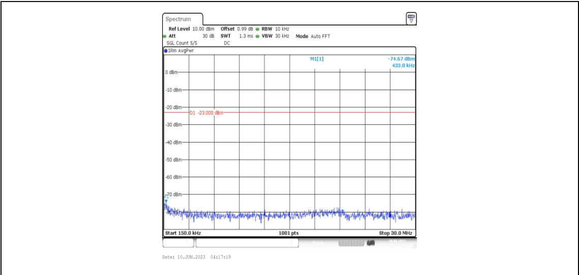
Band12-1.4MHz-16QAM-23017-1RB#0-Range2:0.15~30MHz
