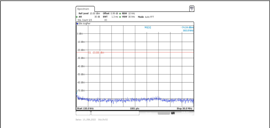
Band12-1.4MHz-QPSK-23173-1RB#0-Range2:0.15~30MHz
