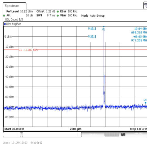
Band12-1.4MHz-QPSK-23017-1RB#0-Range3:30~1000MHz
