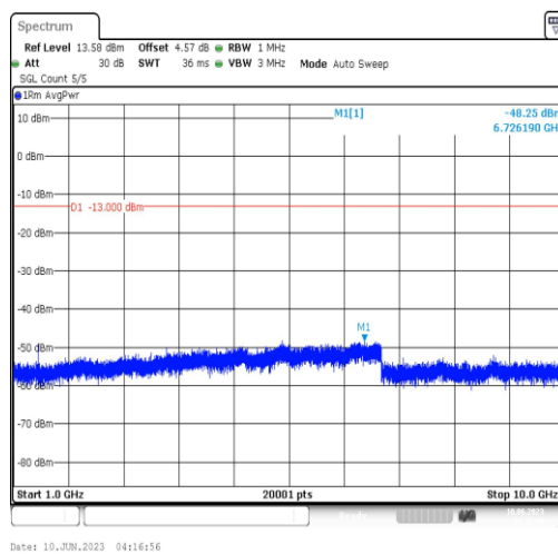
Band12-1.4MHz-QPSK-23017-1RB#0-Range4:1000~10000MHz
