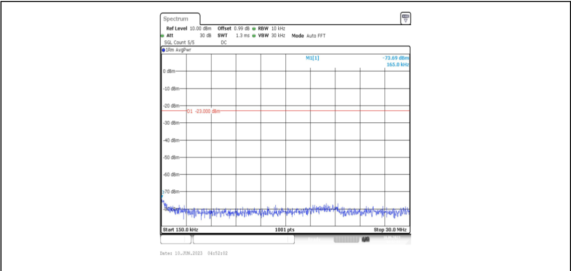
Band12-3MHz-QPSK-23165-1RB#0-Range2:0.15~30MHz
