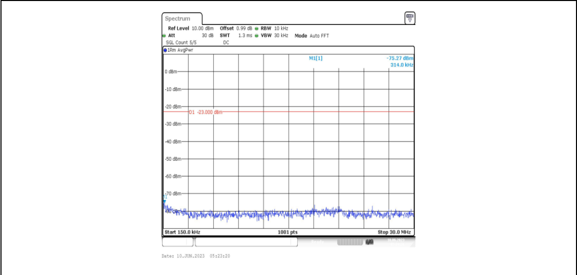
Band12-5MHz-QPSK-23095-1RB#0-Range2:0.15~30MHz
