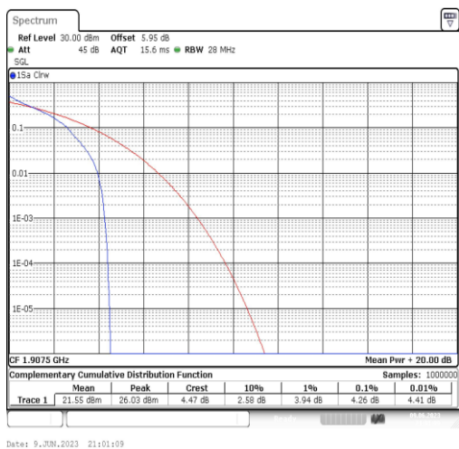
Band2-5MHz-QPSK-19175-1RB#0
