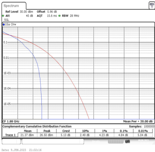
Band2-10MHz-QPSK-18900-1RB#0
