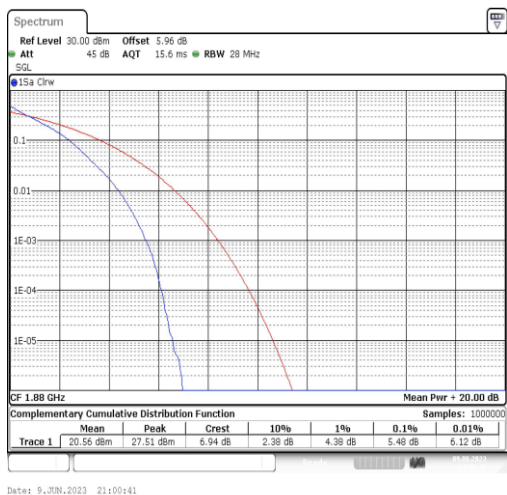
Band2-5MHz-QPSK-18900-25RB#0
