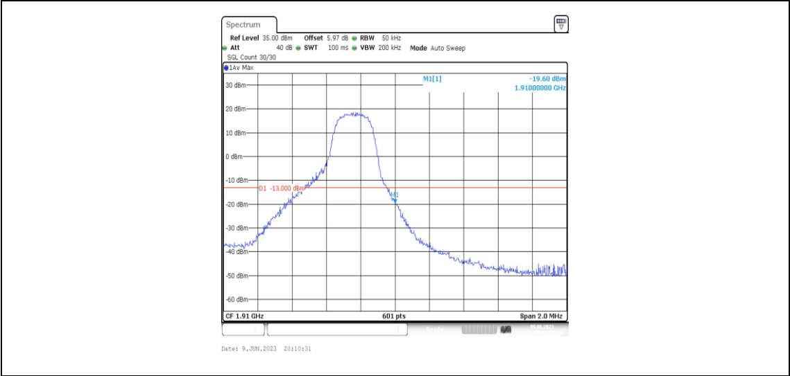
Band2-3MHz-QPSK-19185-1RB#14
