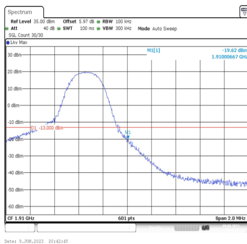
Band2-5MHz-QPSK-19175-1RB#24
