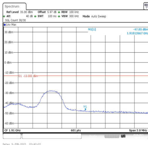
Band2-5MHz-QPSK-19175-1RB#0
