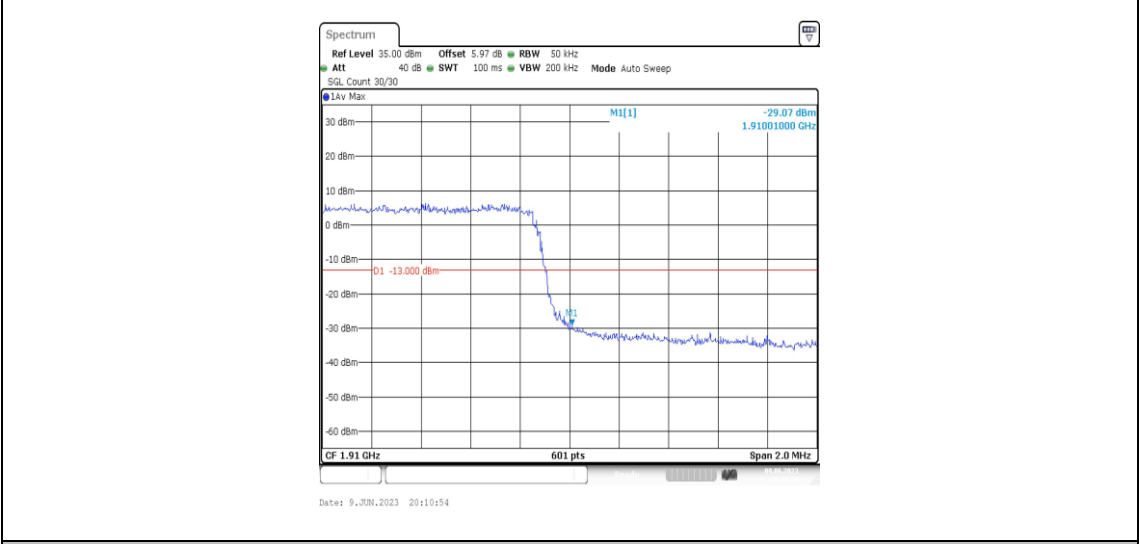
Band2-3MHz-QPSK-19185-15RB#0
