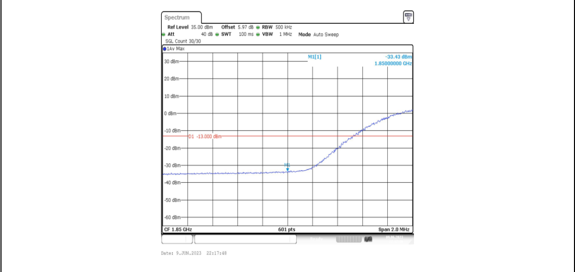
Band2-20MHz-QPSK-18700-100RB#0
