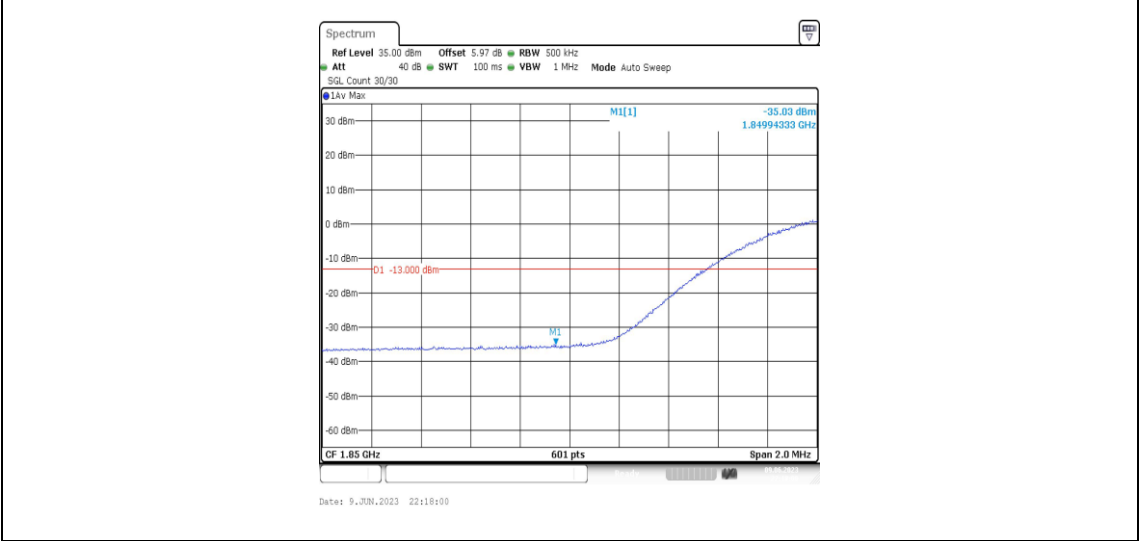
Band2-20MHz-16QAM-18700-100RB#0
