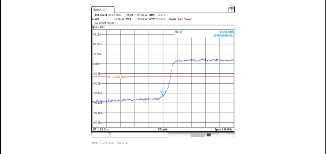
Band2-3MHz-16QAM-18615-15RB#0
