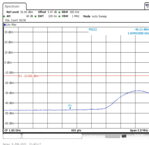
Band2-15MHz-16QAM-18675-1RB#74
