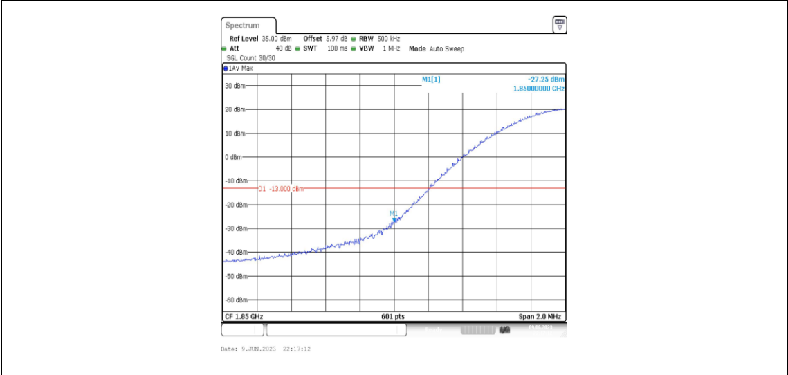
Band2-20MHz-16QAM-18700-1RB#0
