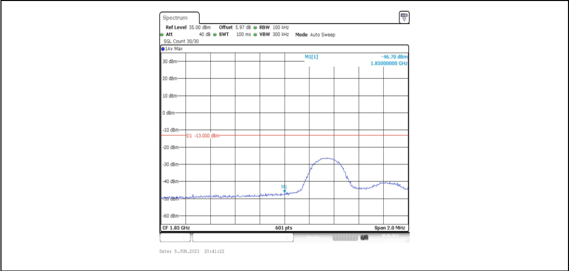
Band2-5MHz-QPSK-18625-1RB#24
