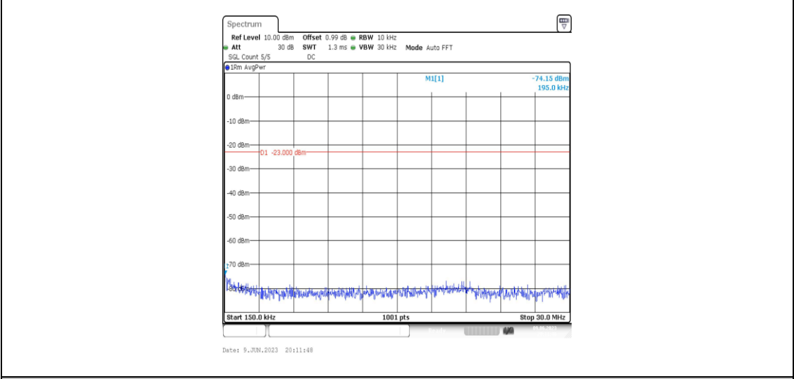
Band2-3MHz-QPSK-18615-1RB#0-Range2:0.15~30MHz
