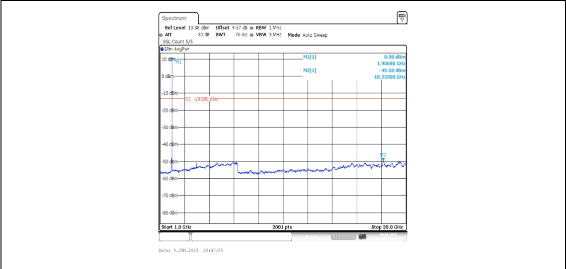
Band2-5MHz-QPSK-19175-1RB#0-Range4:1000~20000MHz
