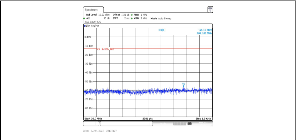
Band2-3MHz-QPSK-19185-1RB#0-Range3:30~1000MHz
