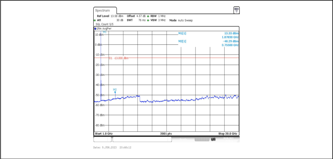
Band2-5MHz-QPSK-18900-1RB#0-Range4:1000~20000MHz
