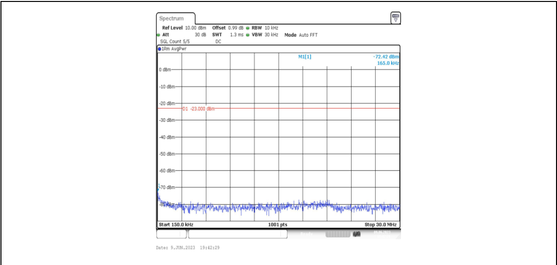
Band2-1.4MHz-QPSK-18900-1RB#0-Range2:0.15~30MHz
