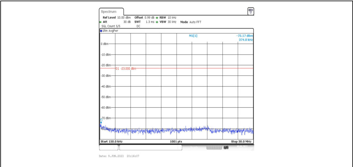
Band2-3MHz-16QAM-19185-1RB#0-Range2:0.15~30MHz
