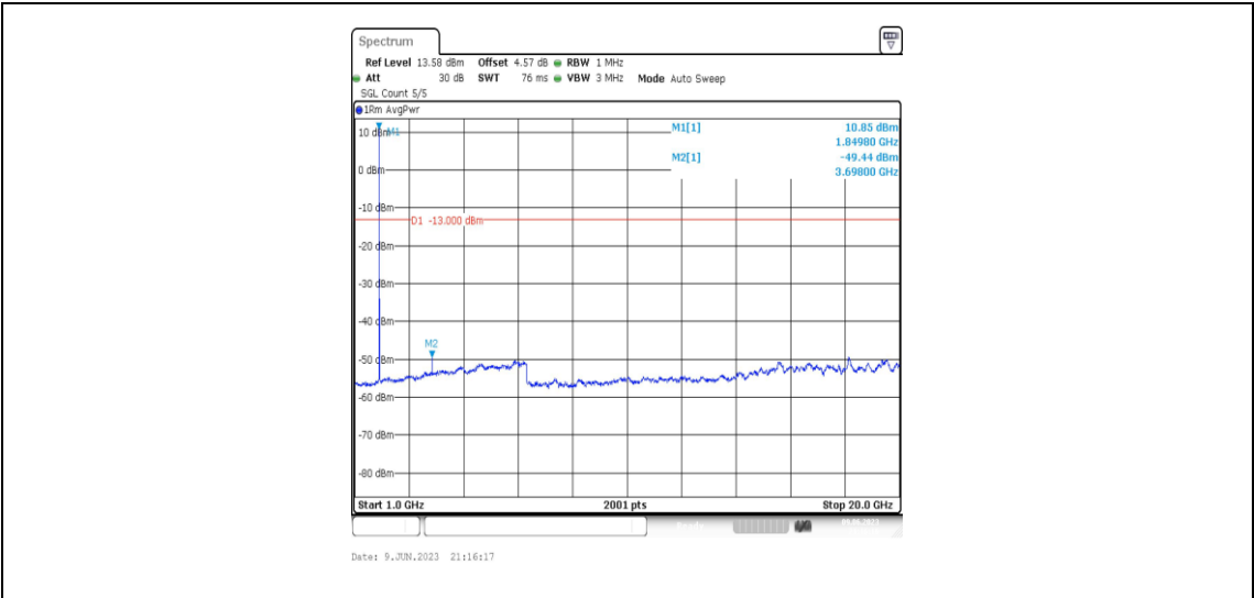
Band2-10MHz-QPSK-18650-1RB#0-Range4:1000~20000MHz
