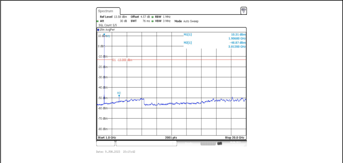
Band2-3MHz-QPSK-19185-1RB#0-Range4:1000~20000MHz
