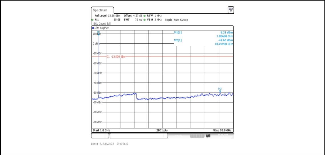
Band2-3MHz-16QAM-19185-1RB#0-Range4:1000~20000MHz
