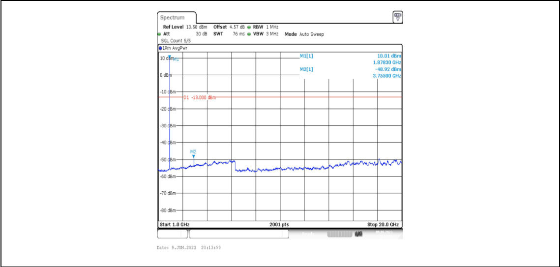
Band2-3MHz-QPSK-18900-1RB#0-Range4:1000~20000MHz
