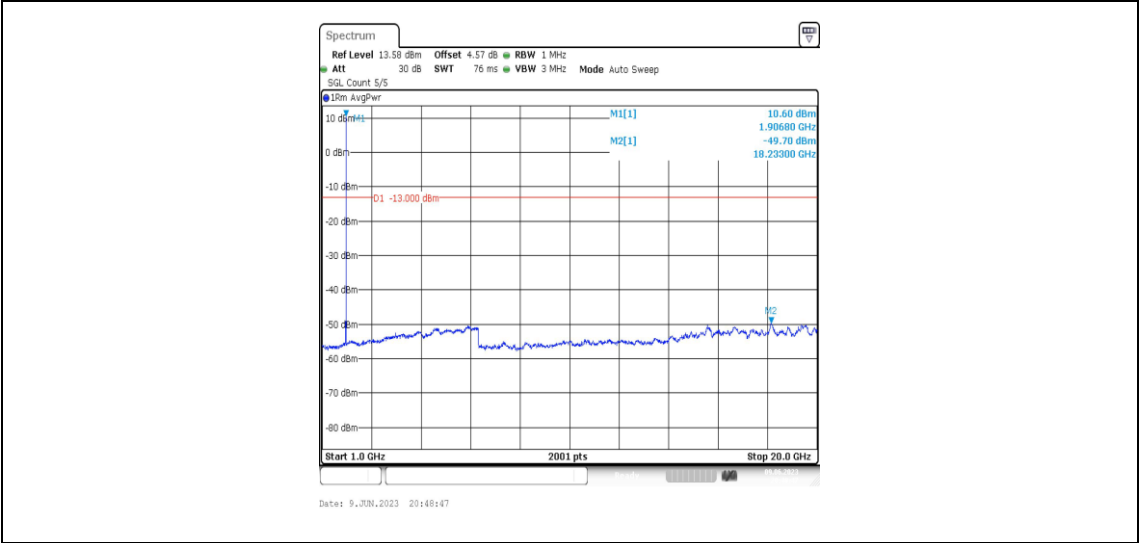
Band2-5MHz-16QAM-19175-1RB#0-Range4:1000~20000MHz
