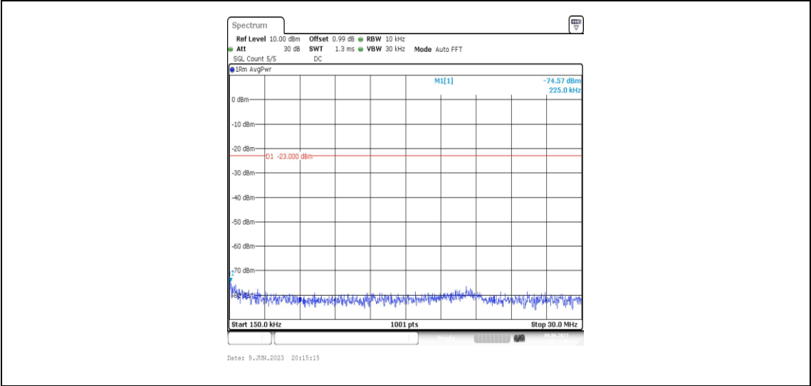
Band2-3MHz-QPSK-19185-1RB#0-Range2:0.15~30MHz
