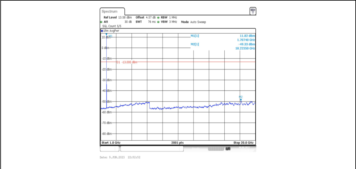
Band4-1.4MHz-QPSK-19957-1RB#0-Range4:1000~20000MHz
