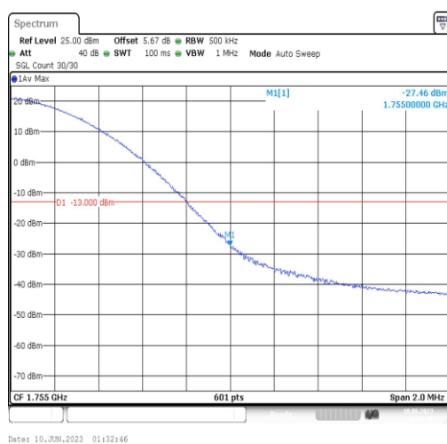
Band4-20MHz-QPSK-20300-1RB#99
