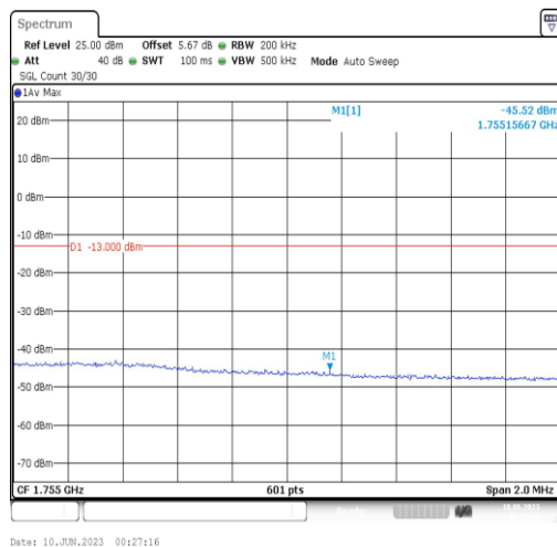
Band4-10MHz-QPSK-20350-1RB#0
