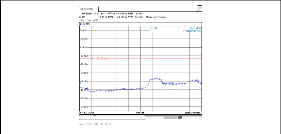
Band4-3MHz-QPSK-19965-1RB#14
