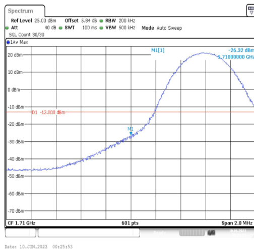
Band4-10MHz-QPSK-20000-1RB#0
