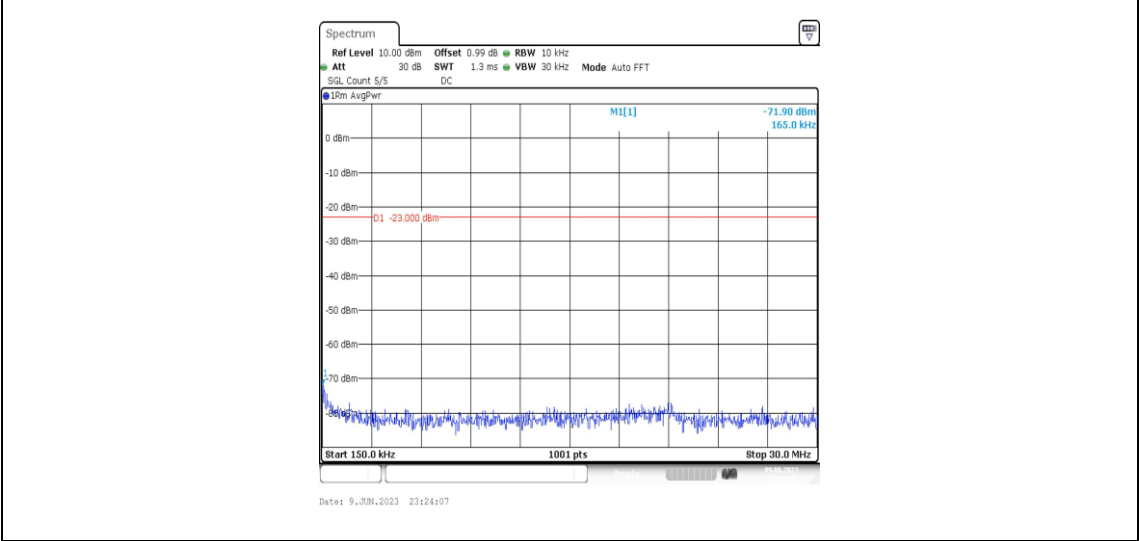
Band4-3MHz-QPSK-19965-1RB#0-Range2:0.15~30MHz
