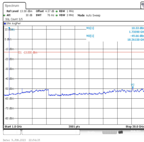
Band4-1.4MHz-QPSK-20175-1RB#0-Range4:1000~20000MHz
