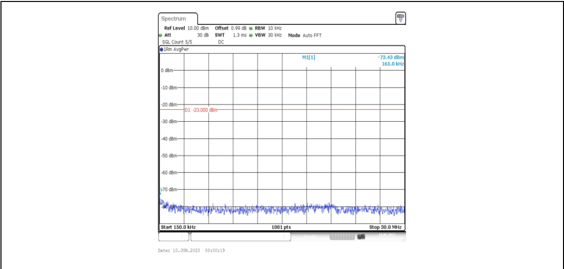
Band4-5MHz-QPSK-20375-1RB#0-Range2:0.15~30MHz
