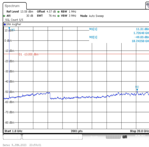
Band4-5MHz-QPSK-20175-1RB#0-Range4:1000~20000MHz
