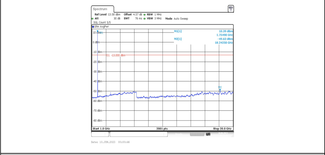
Band4-5MHz-QPSK-20375-1RB#0-Range4:1000~20000MHz
