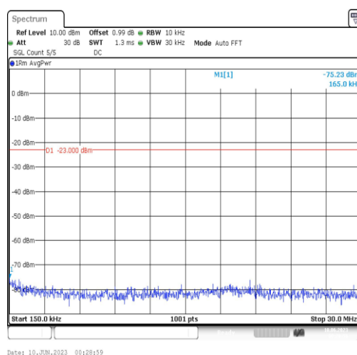
Band4-10MHz-QPSK-20000-1RB#0-Range2:0.15~30MHz
