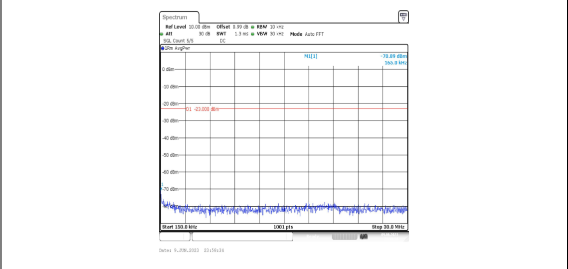
Band4-5MHz-QPSK-20175-1RB#0-Range2:0.15~30MHz
