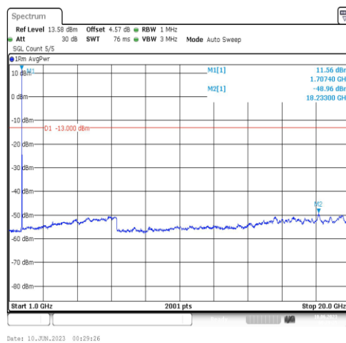
Band4-10MHz-QPSK-20000-1RB#0-Range4:1000~20000MHz
