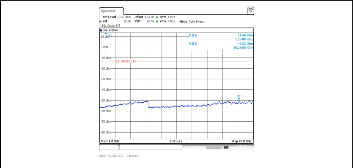
Band4-3MHz-QPSK-20385-1RB#0-Range4:1000~20000MHz
