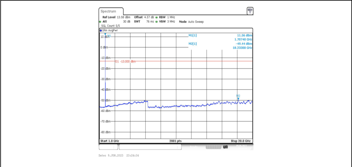
Band4-3MHz-QPSK-19965-1RB#0-Range4:1000~20000MHz
