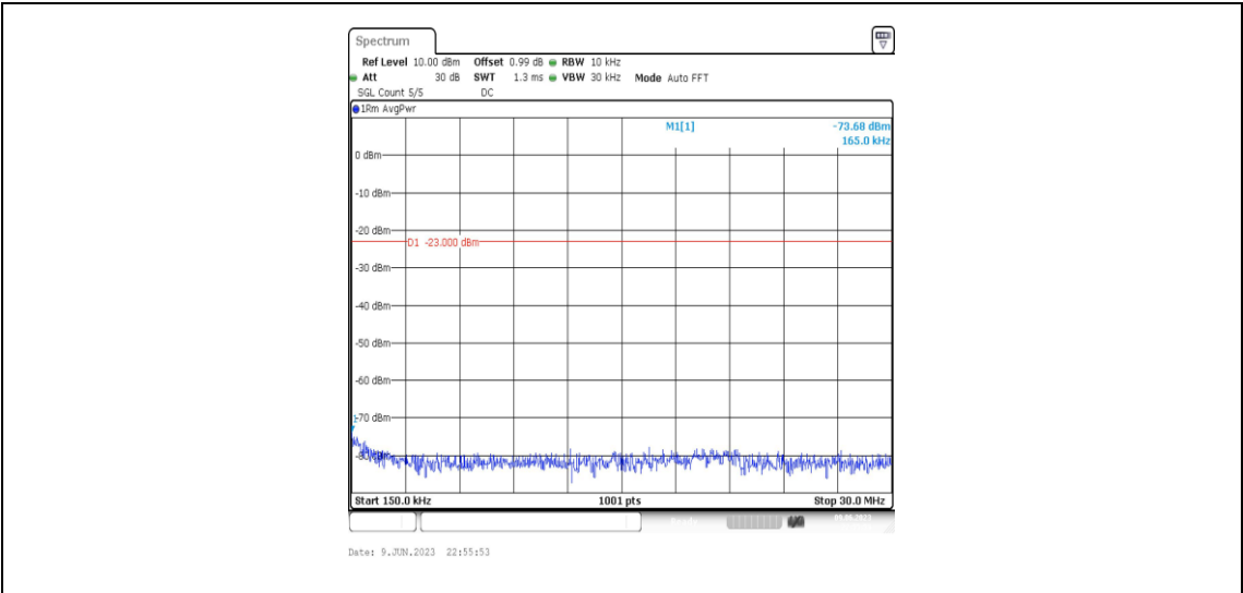
Band4-1.4MHz-QPSK-20393-1RB#0-Range2:0.15~30MHz
