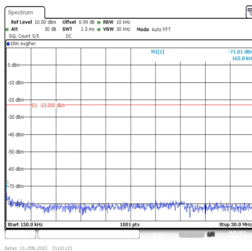
Band4-15MHz-QPSK-20025-1RB#0-Range2:0.15~30MHz
