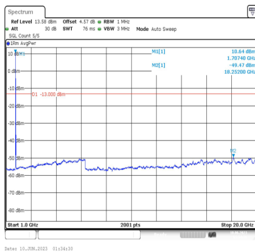
Band4-20MHz-QPSK-20050-1RB#0-Range4:1000~20000MHz
