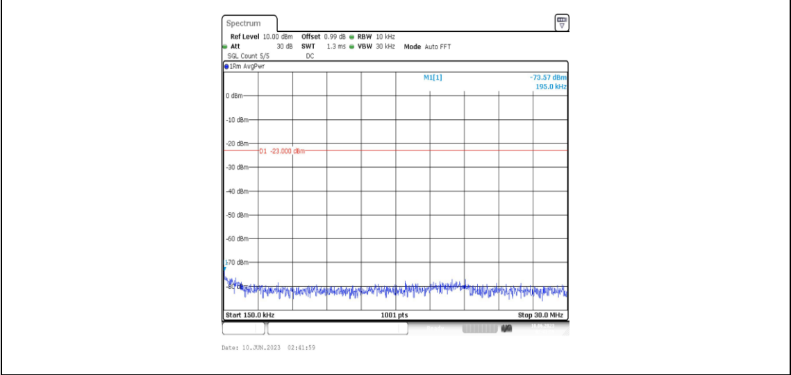
Band5-3MHz-QPSK-20635-1RB#0-Range2:0.15~30MHz
