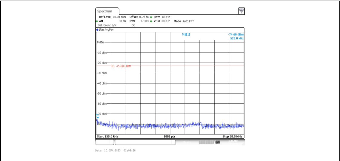
Band5-1.4MHz-QPSK-20525-1RB#0-Range2:0.15~30MHz
