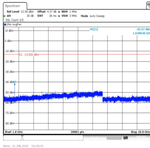
Band5-3MHz-QPSK-20415-1RB#0-Range4:1000~10000MHz
