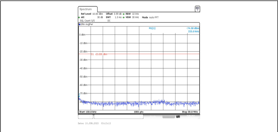
Band5-5MHz-QPSK-20525-1RB#0-Range2:0.15~30MHz
