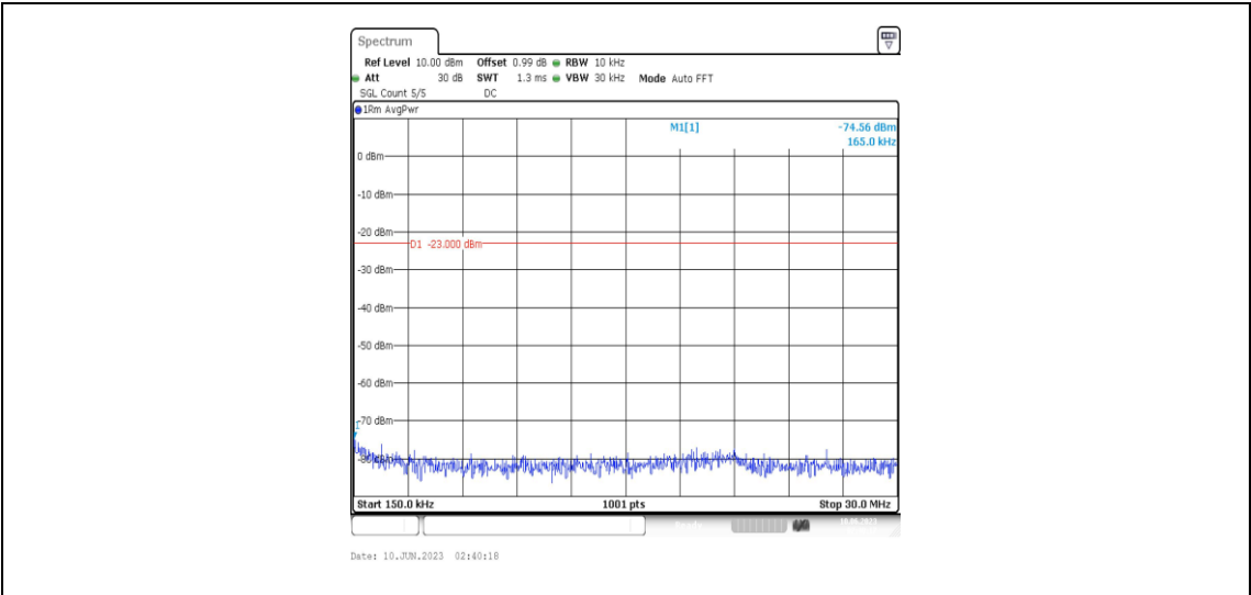
Band5-3MHz-QPSK-20525-1RB#0-Range2:0.15~30MHz
