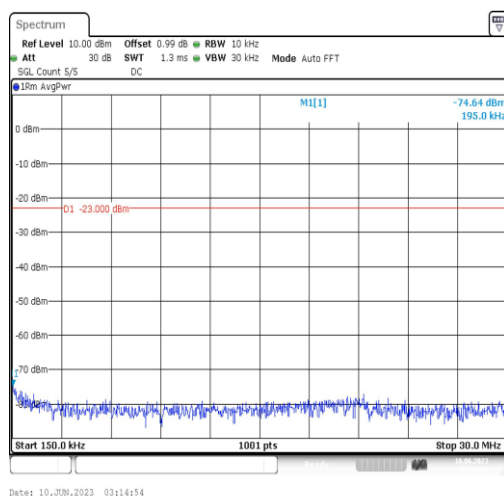
Band5-5MHz-QPSK-20625-1RB#0-Range2:0.15~30MHz
