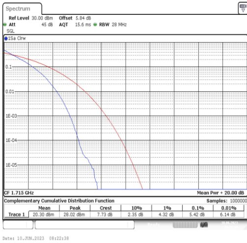
Band66-10MHz-QPSK-132022-50RB#0
