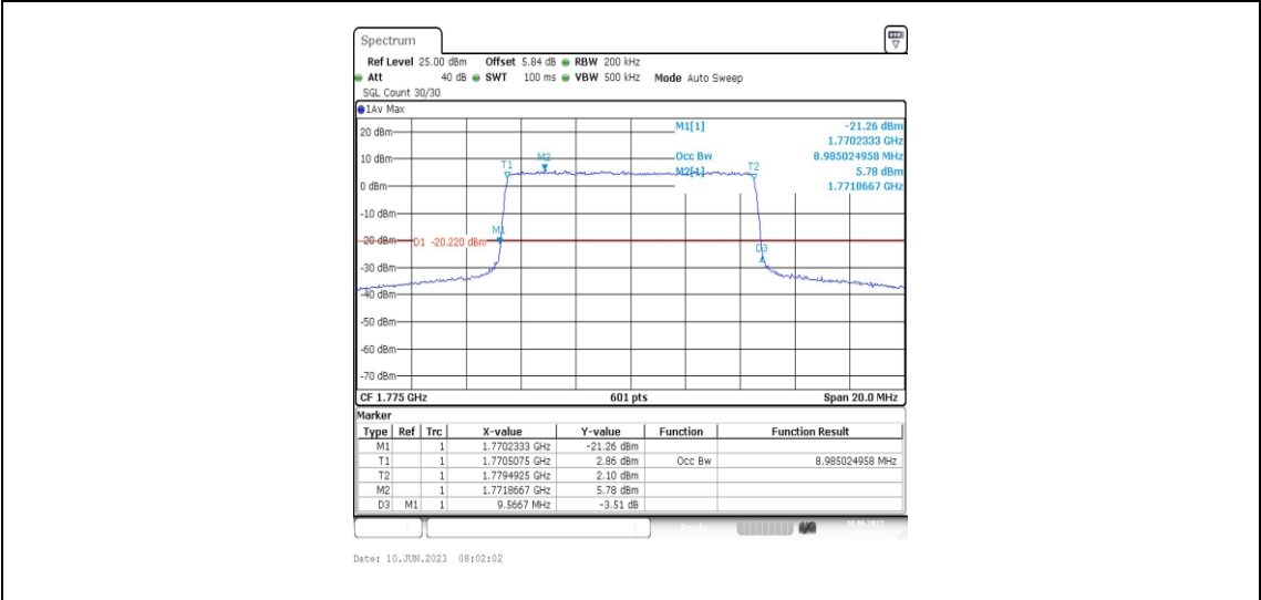
Band66-10MHz-QPSK-132622-50RB#0-8.985
