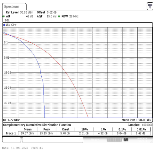
Band66-20MHz-QPSK-132072-1RB#0
