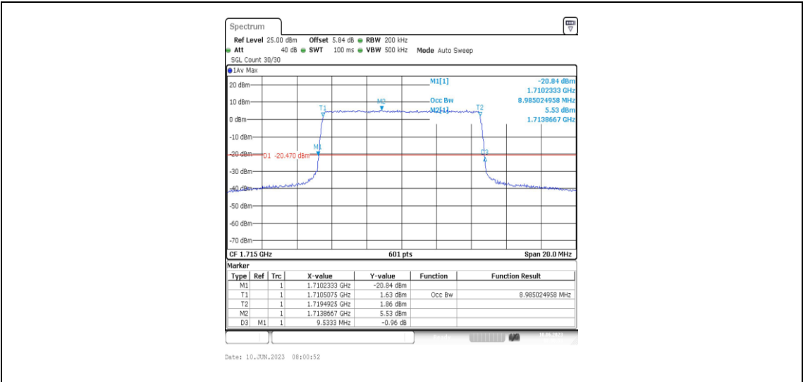
Band66-10MHz-QPSK-132022-50RB#0-8.985
