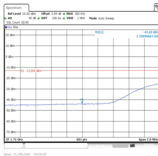
Band66-20MHz-QPSK-132072-1RB#99
