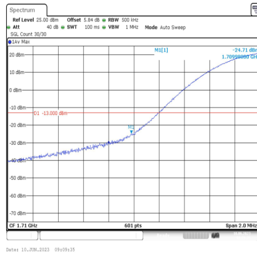
Band66-20MHz-QPSK-132072-1RB#0
