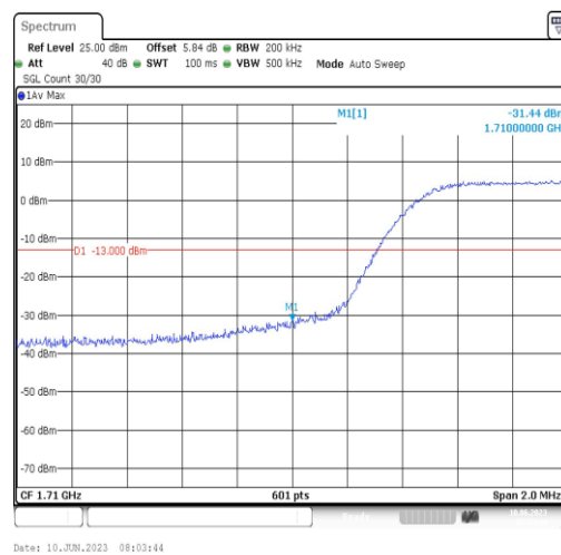
Band66-10MHz-QPSK-132022-50RB#0
