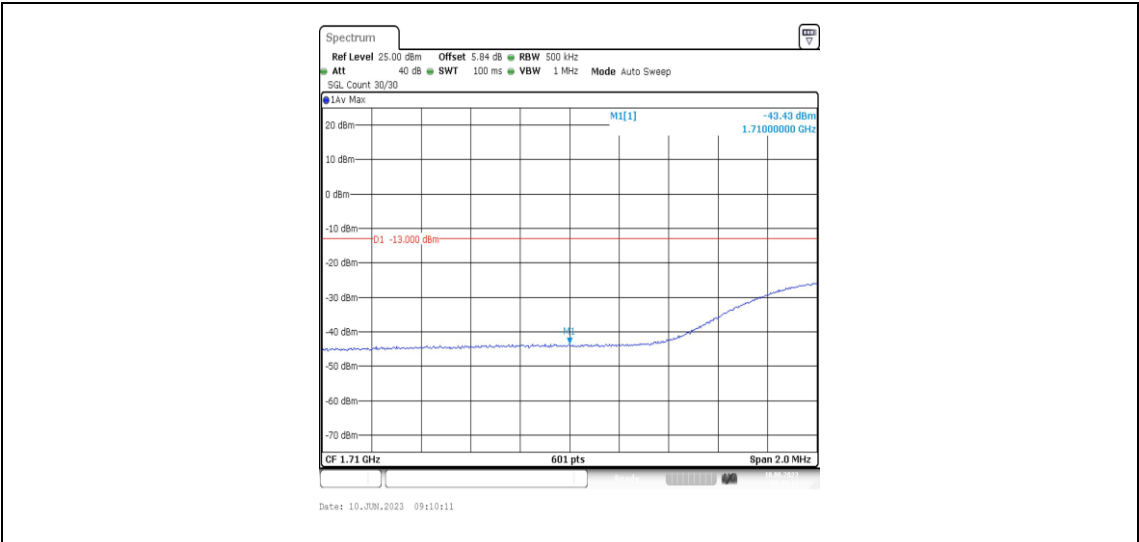
Band66-20MHz-16QAM-132072-1RB#99
