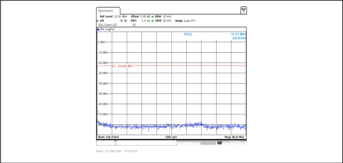
Band66-5MHz-QPSK-131997-1RB#0-Range2:0.15~30MHz
