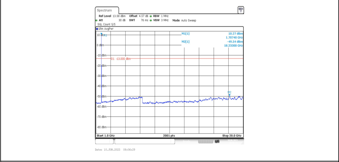
Band66-10MHz-QPSK-132022-1RB#0-Range4:1000~20000MHz
