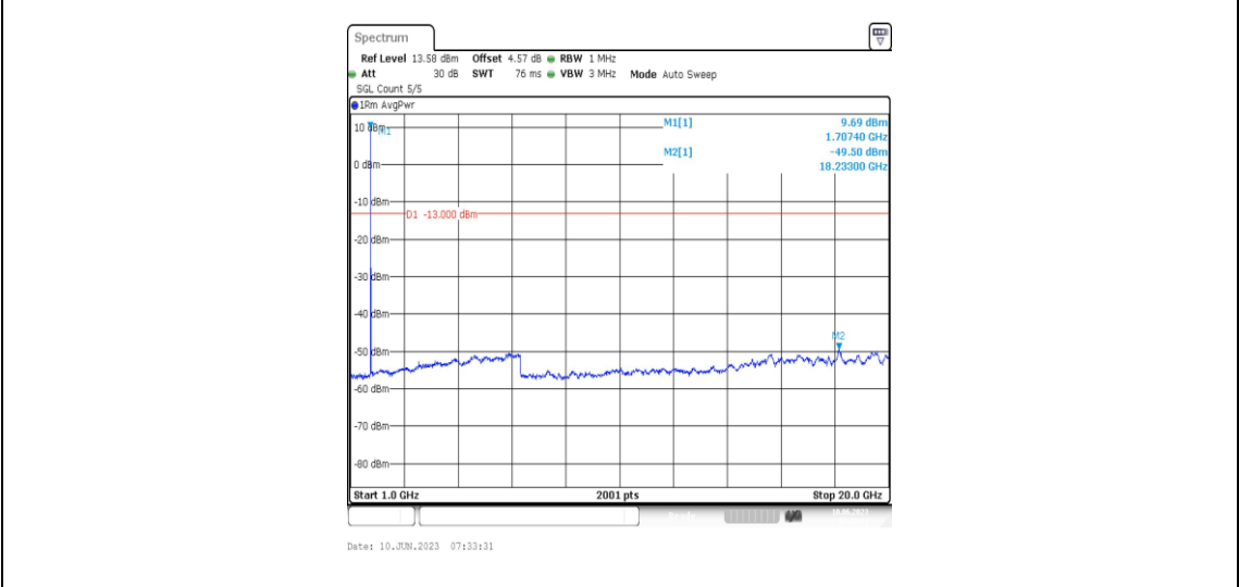
Band66-5MHz-QPSK-131997-1RB#0-Range4:1000~20000MHz
