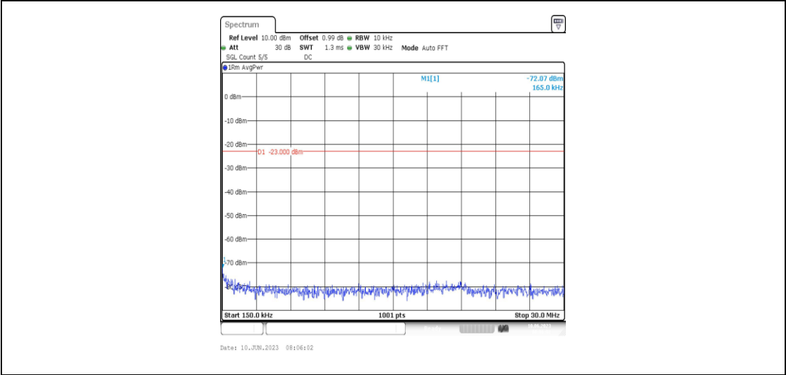
Band66-10MHz-QPSK-132022-1RB#0-Range2:0.15~30MHz
