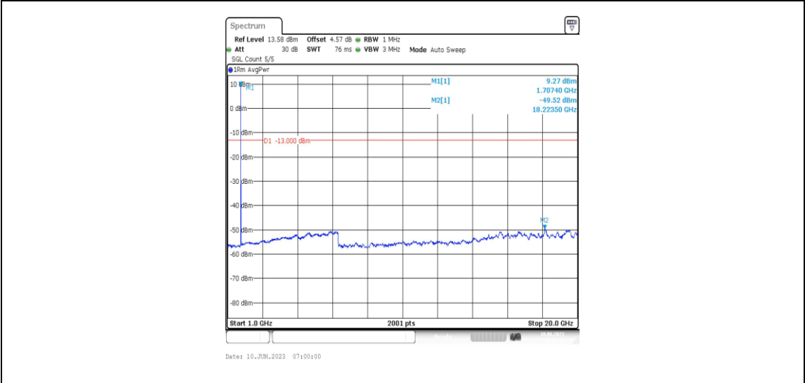
Band66-3MHz-QPSK-131987-1RB#0-Range4:1000~20000MHz
