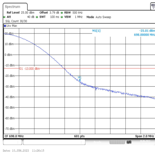
Band71-20MHz-16QAM-133372-1RB#99
