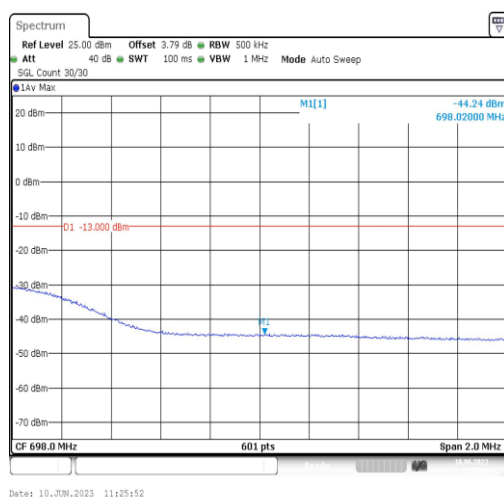
Band71-20MHz-16QAM-133372-1RB#0
