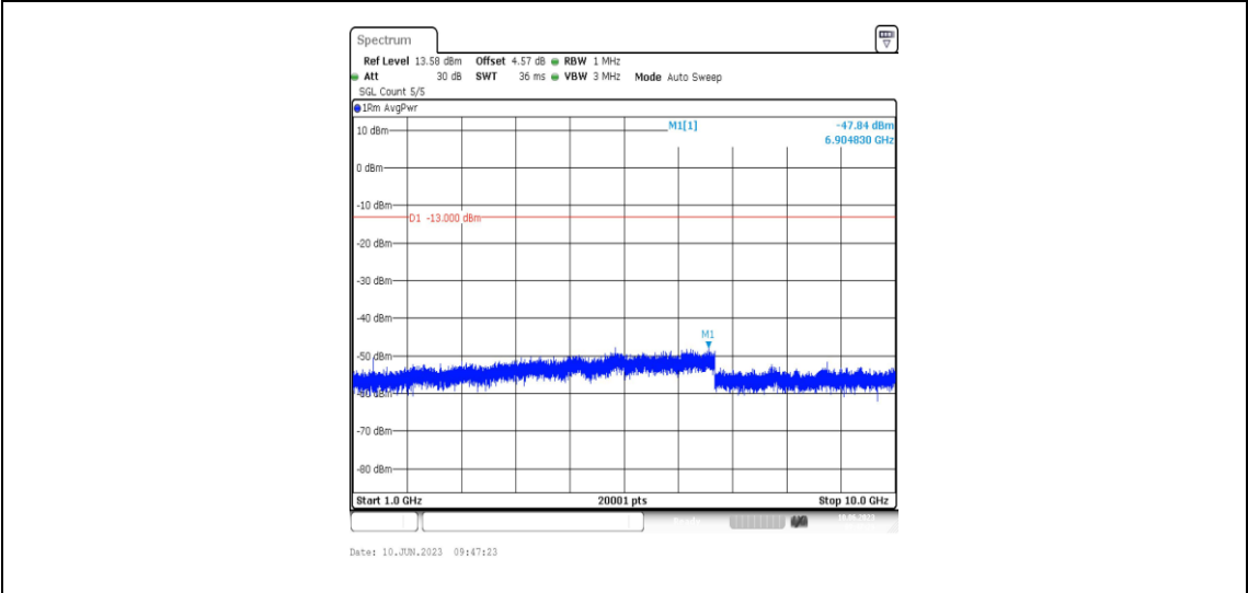
Band71-5MHz-QPSK-133147-1RB#0-Range4:1000~10000MHz
