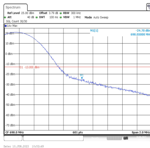
Band71-15MHz-QPSK-133397-1RB#74
