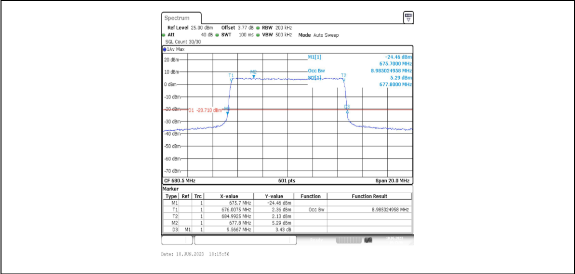
Band71-10MHz-QPSK-133297-50RB#0-8.985
