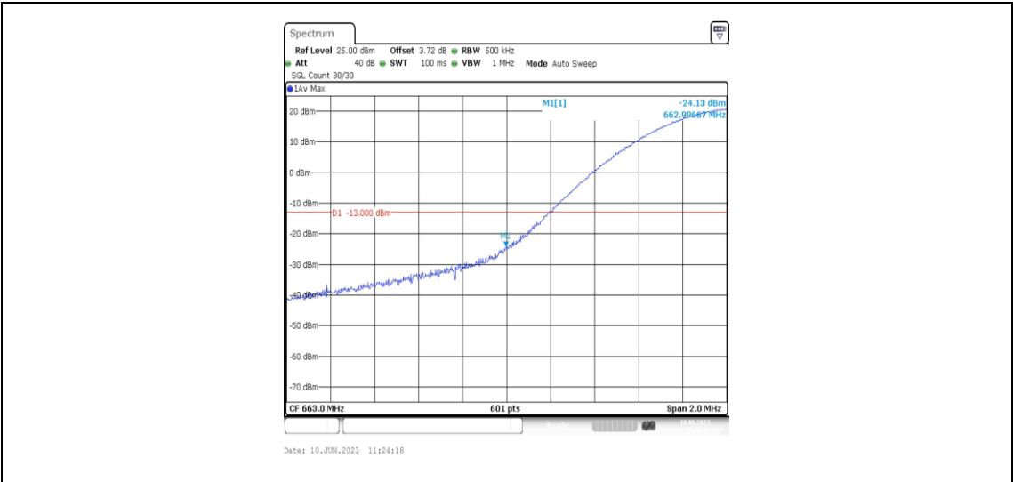
Band71-20MHz-QPSK-133222-1RB#0
