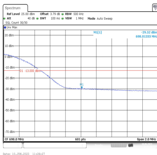
Band71-20MHz-QPSK-133372-100RB#0
