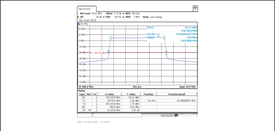
Band71-20MHz-QPSK-133372-100RB#0-18.037
