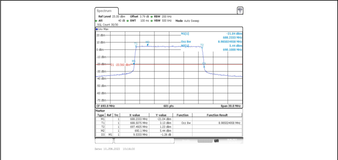
Band71-10MHz-QPSK-133422-50RB#0-8.985
