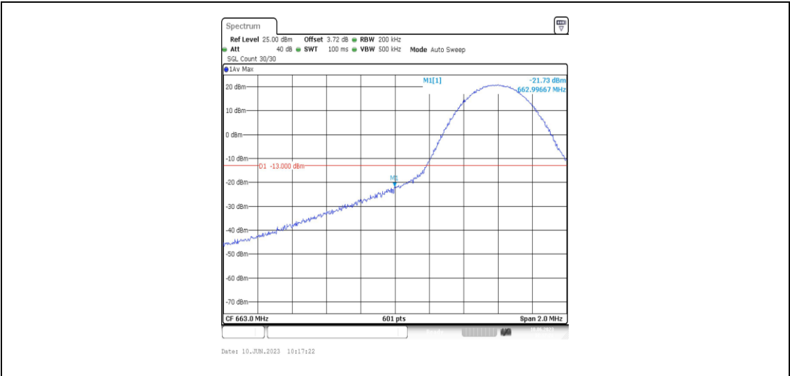
Band71-10MHz-QPSK-133172-1RB#0
