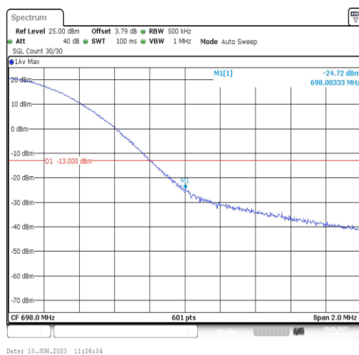
Band71-20MHz-QPSK-133372-1RB#99
