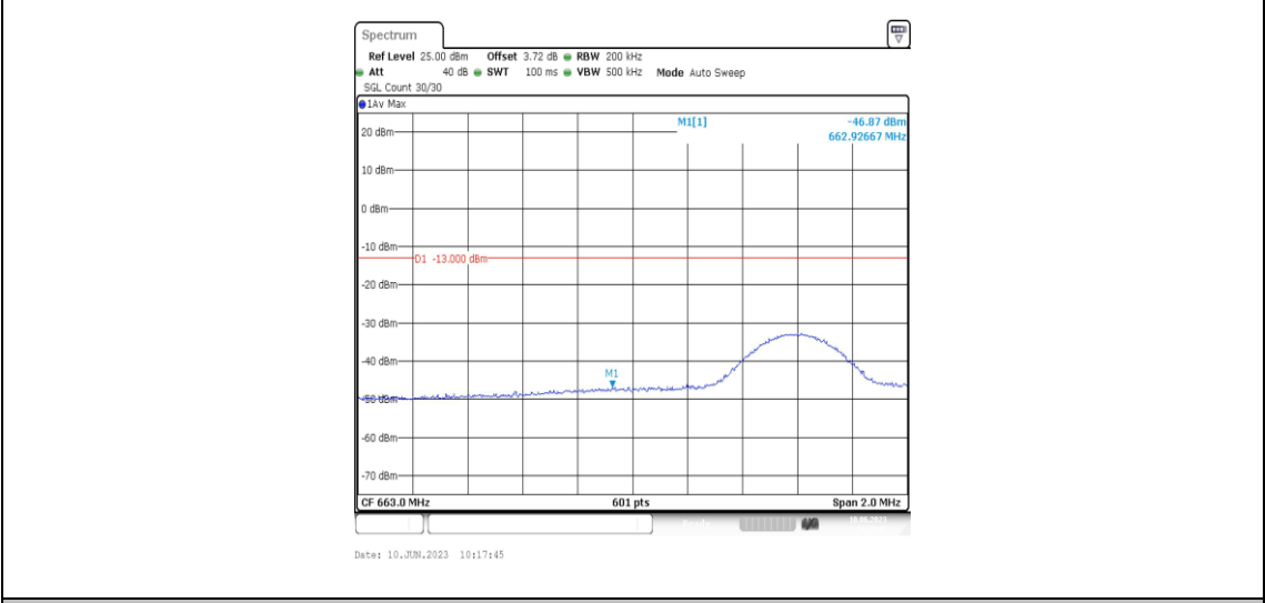
Band71-10MHz-QPSK-133172-1RB#49
