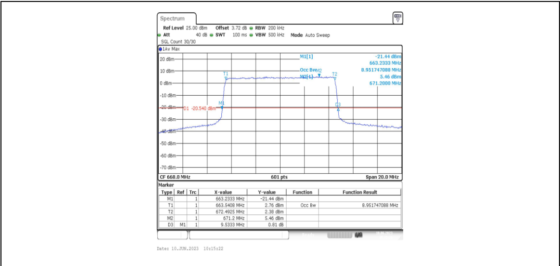
Band71-10MHz-QPSK-133172-50RB#0-8.952
