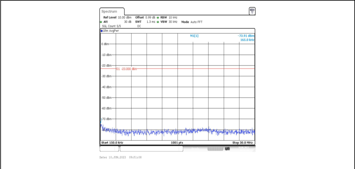
Band71-5MHz-16QAM-133447-1RB#0-Range2:0.15~30MHz
