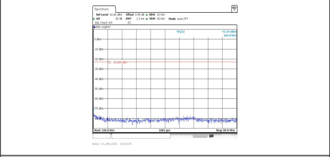
Band71-15MHz-QPSK-133197-1RB#0-Range2:0.15~30MHz
