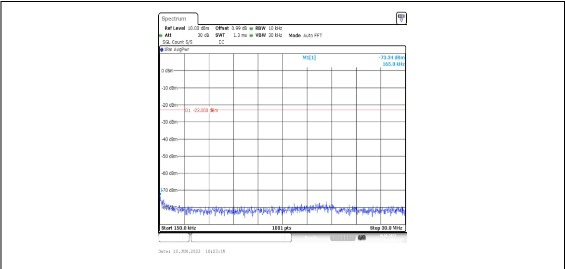
Band71-10MHz-QPSK-133422-1RB#0-Range2:0.15~30MHz
