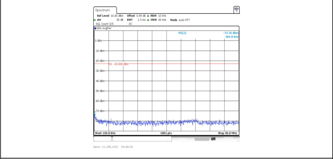
Band71-5MHz-QPSK-133297-1RB#0-Range2:0.15~30MHz
