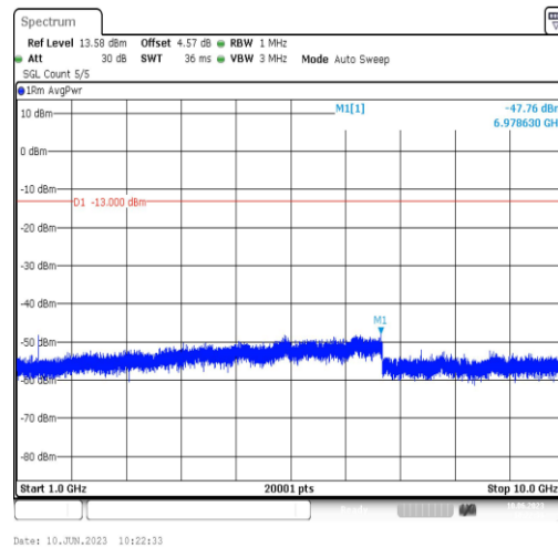
Band71-10MHz-QPSK-133297-1RB#0-Range4:1000~10000MHz
