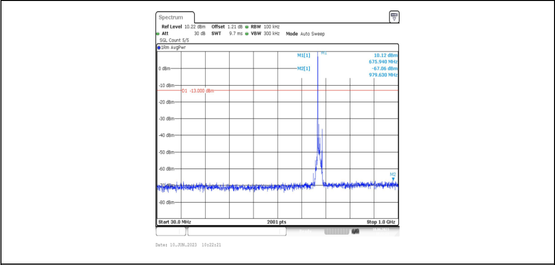
Band71-10MHz-QPSK-133297-1RB#0-Range3:30~1000MHz
