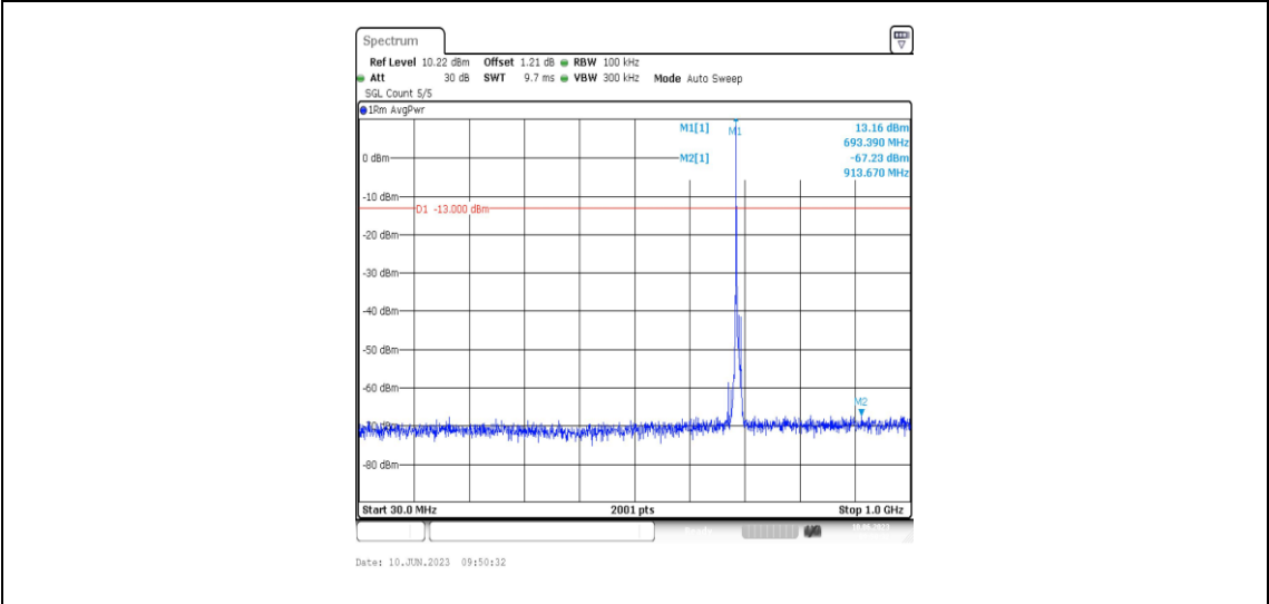
Band71-5MHz-QPSK-133447-1RB#0-Range3:30~1000MHz
