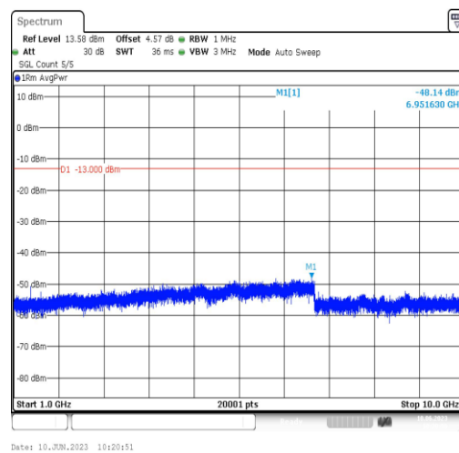
Band71-10MHz-QPSK-133172-1RB#0-Range4:1000~10000MHz
