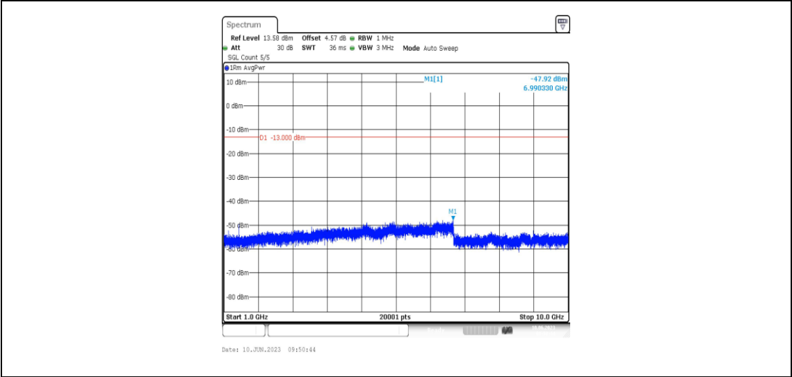
Band71-5MHz-QPSK-133447-1RB#0-Range4:1000~10000MHz
