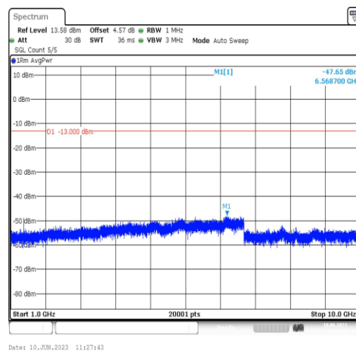
Band71-20MHz-QPSK-133222-1RB#0-Range4:1000~10000MHz
