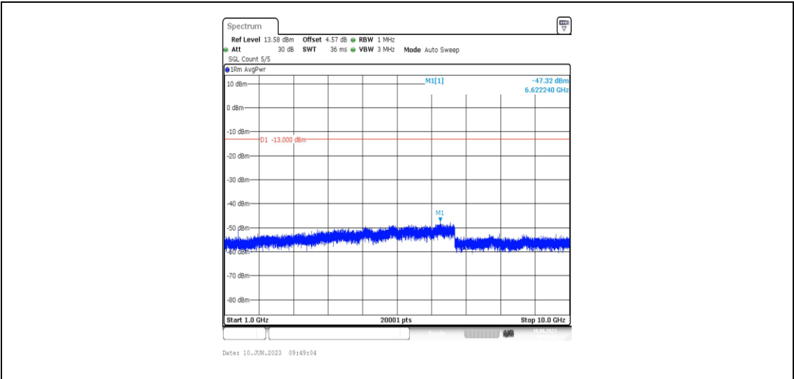
Band71-5MHz-QPSK-133297-1RB#0-Range4:1000~10000MHz
