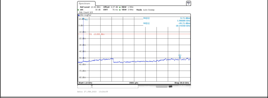
Band2-3MHz-16QAM-19185-1RB#0-Range4:1000~20000MHz
