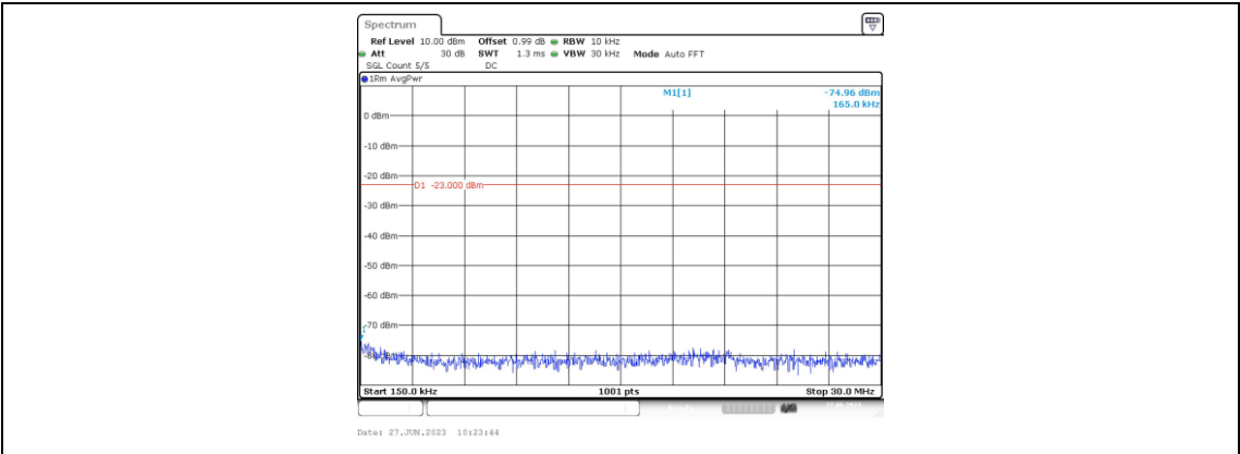
Band2-3MHz-16QAM-19185-1RB#0-Range2:0.15~30MHz
