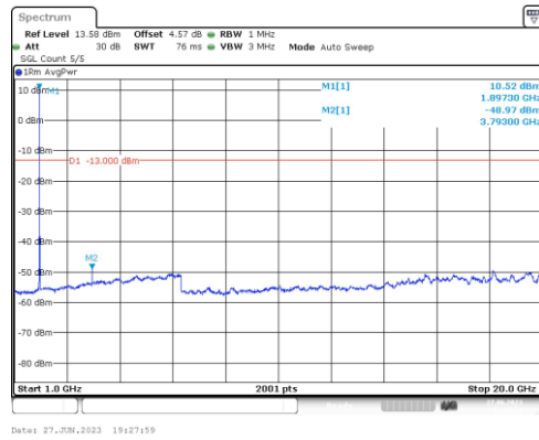
Band2-15MHz-QPSK-19125-1RB#0-Range4:1000~20000MHz
