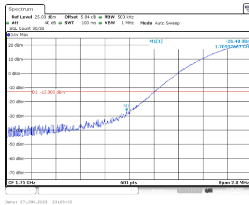
Band4-20MHz-QPSK-20050-1RB#0
