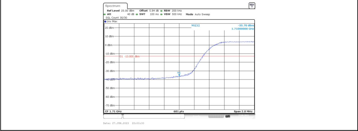
Band4-10MHz-QPSK-20000-50RB#0
