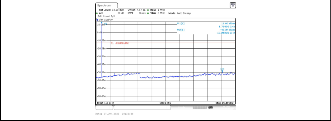
Band4-1.4MHz-QPSK-20393-1RB#0-Range4:1000~20000MHz
