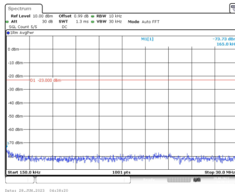
Band66-3MHz-QPSK-131987-1RB#0-Range2:0.15~30MHz
