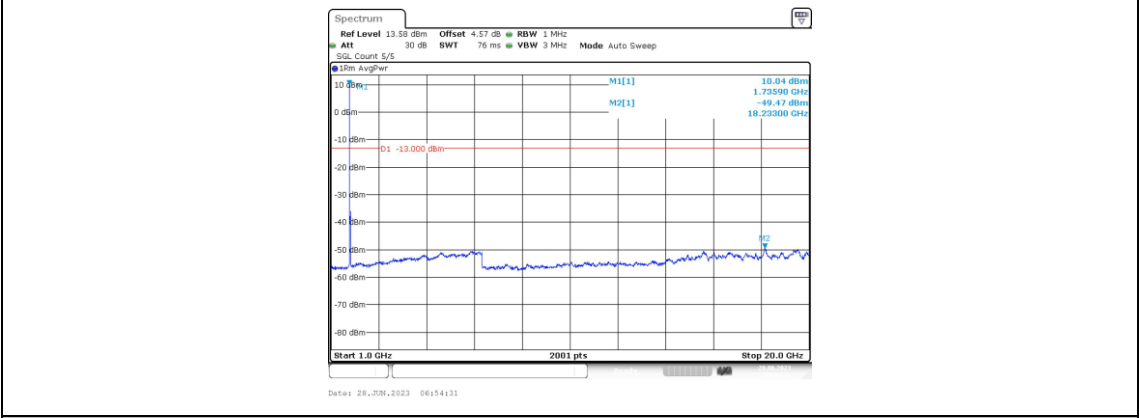
Band66-20MHz-QPSK-132322-1RB#0-Range4:1000~20000MHz
