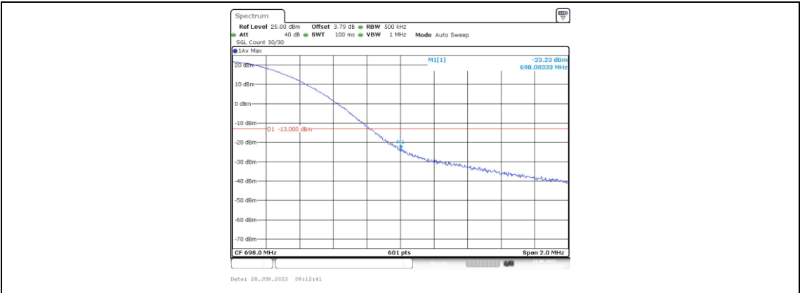
Band71-20MHz-QPSK-133372-1RB#99
