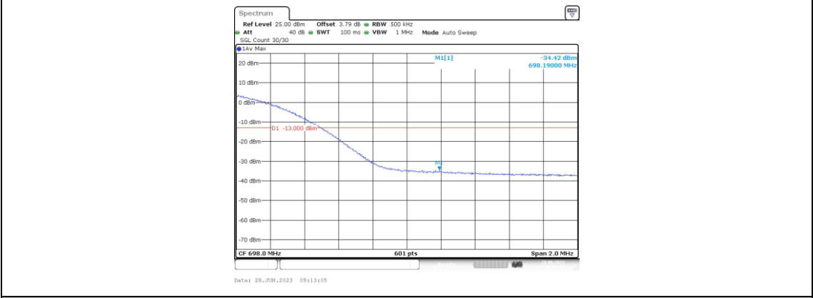
Band71-20MHz-QPSK-133372-100RB#0
