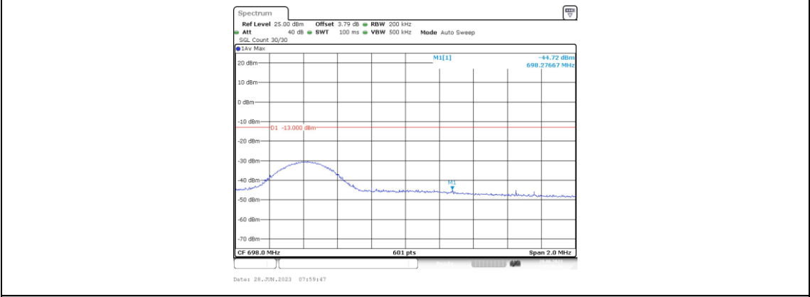
Band71-10MHz-QPSK-133422-1RB#0
