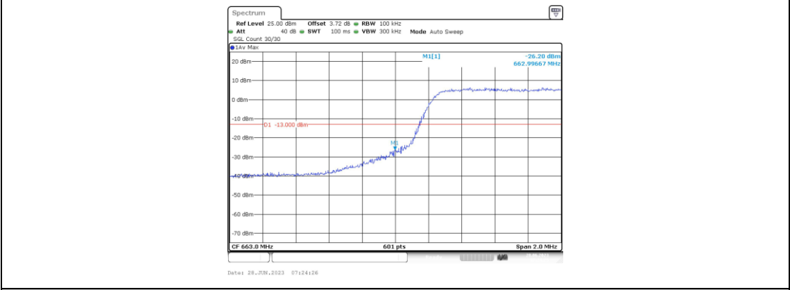
Band71-5MHz-QPSK-133147-25RB#0
