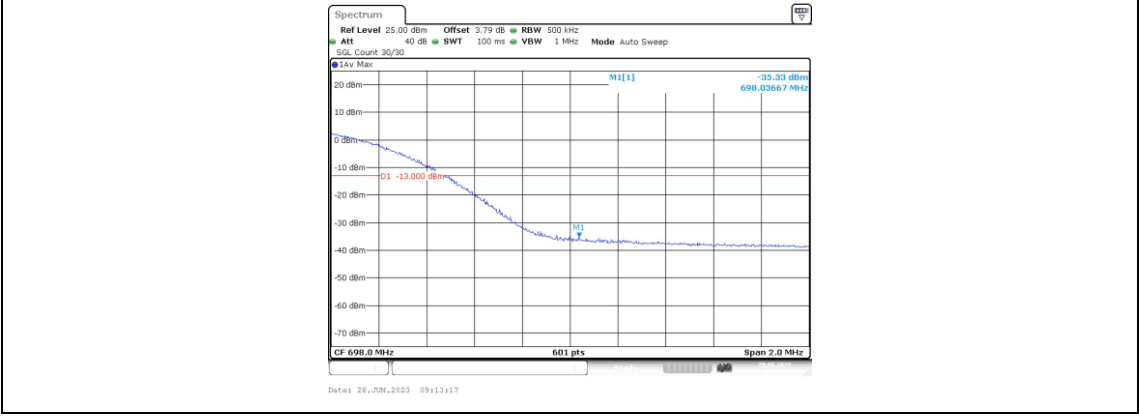
Band71-20MHz-QPSK-133372-100RB#0
