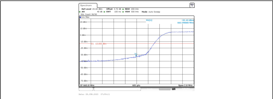
Band71-10MHz-QPSK-133172-50RB#0
