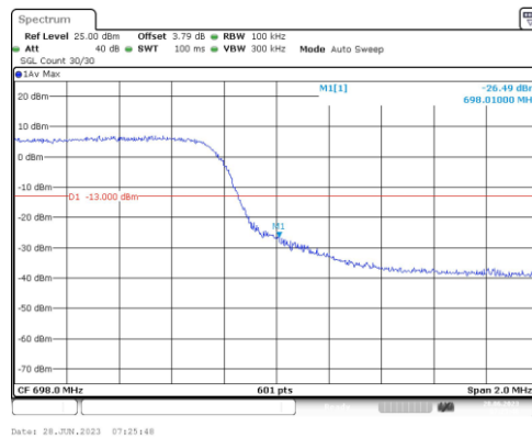
Band71-5MHz-QPSK-133447-25RB#0
