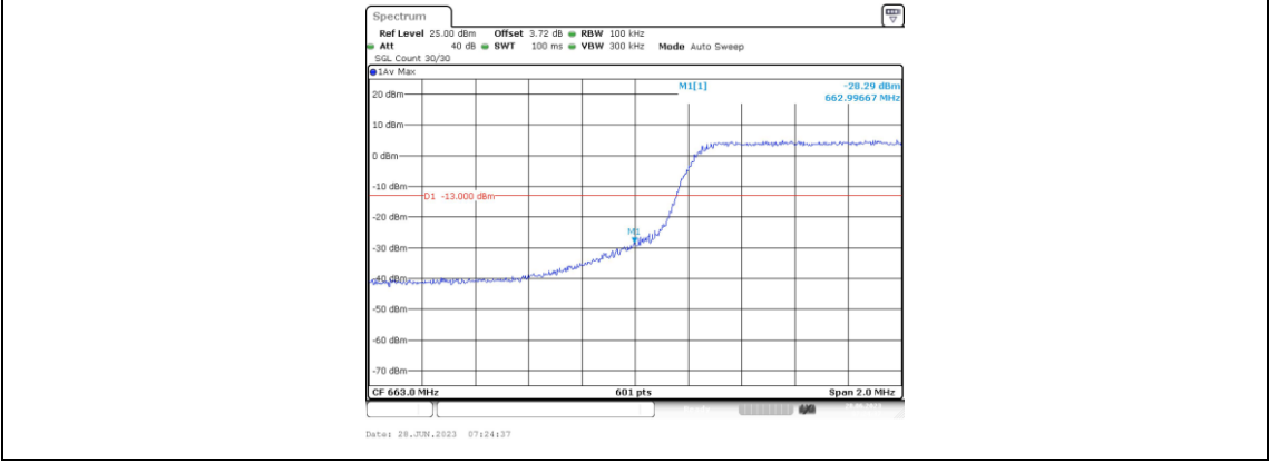
Band71-5MHz-QPSK-133147-25RB#0
