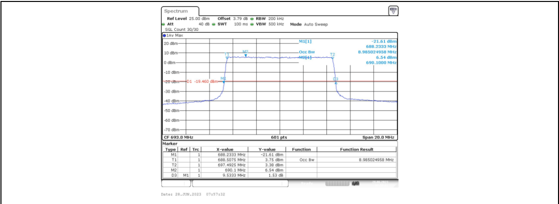
Band71-10MHz-QPSK-133422-50RB#0-8.985
