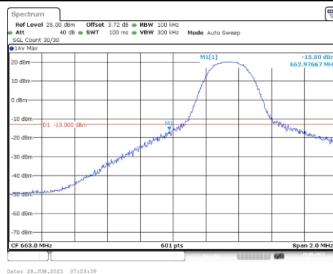
Band71-5MHz-QPSK-133147-1RB#0
